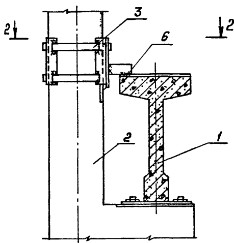
Рис. 5.36. Усиление крепления подкрановой балки к колонне
