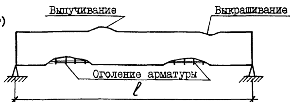
Рис. I. Дефекты железобетонных балок
