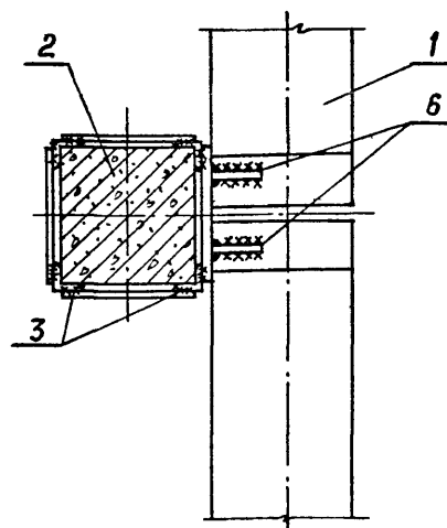
Рис. 5.36. Усиление крепления подкрановой балки к колонне
