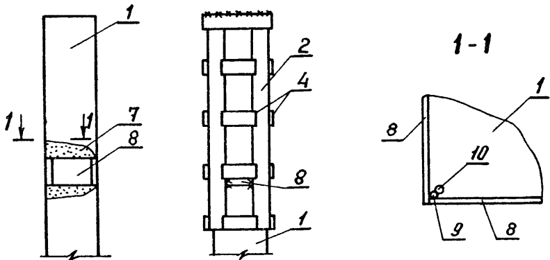
Рис. 4.14. Усиление железобетонных колонн стальной облоймой
