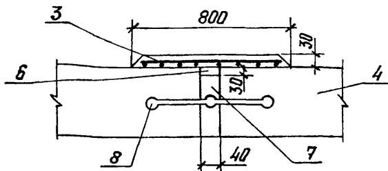
Рис. 5.3. Ремонт железобетонных емкостей
