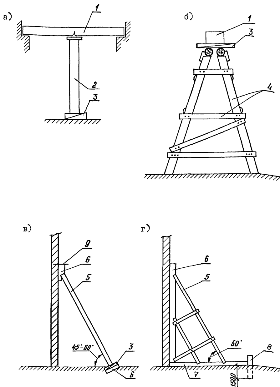
Рис. 4.17. Временные крепления поврежденных конструкций а - в виде стоек; б - пространственной опоры; в, г - подкосов для стен; 1 - конструкция; 2 - временная подпорка-стойка из бревна; 3 - клинья; 4 - пространственная опора; 5 - подкосы из бревен \varnothing 16-20 см; 6 - прокладка диаметром 16-20 см; 7 - лежень диаметром 18-22 см; 8 - упорный столб диаметром 18-22 см; 9 - крепежный штырь.
