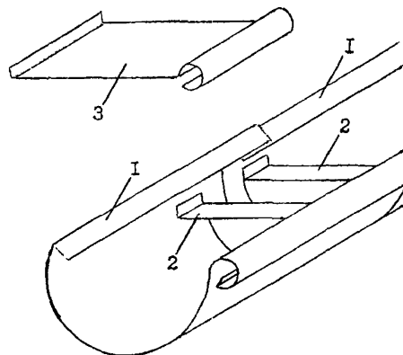
Рис.29. Скользящие соединения шва на стыке полукруглых желобов 1 – полукруглый желоб; 2 – ограничитель; 3 – покрывная полоса.
