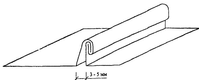
Рис.5 Компенсационный стык
