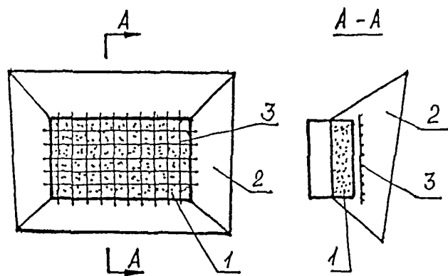
Рис. 1а. Схема “светлого” газового инфракрасного излучателя
