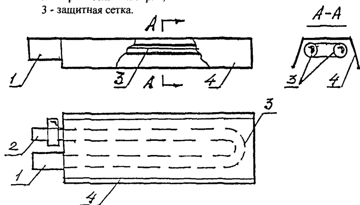
Рис. 1б. Схема “темного” газового инфракрасного излучателя
