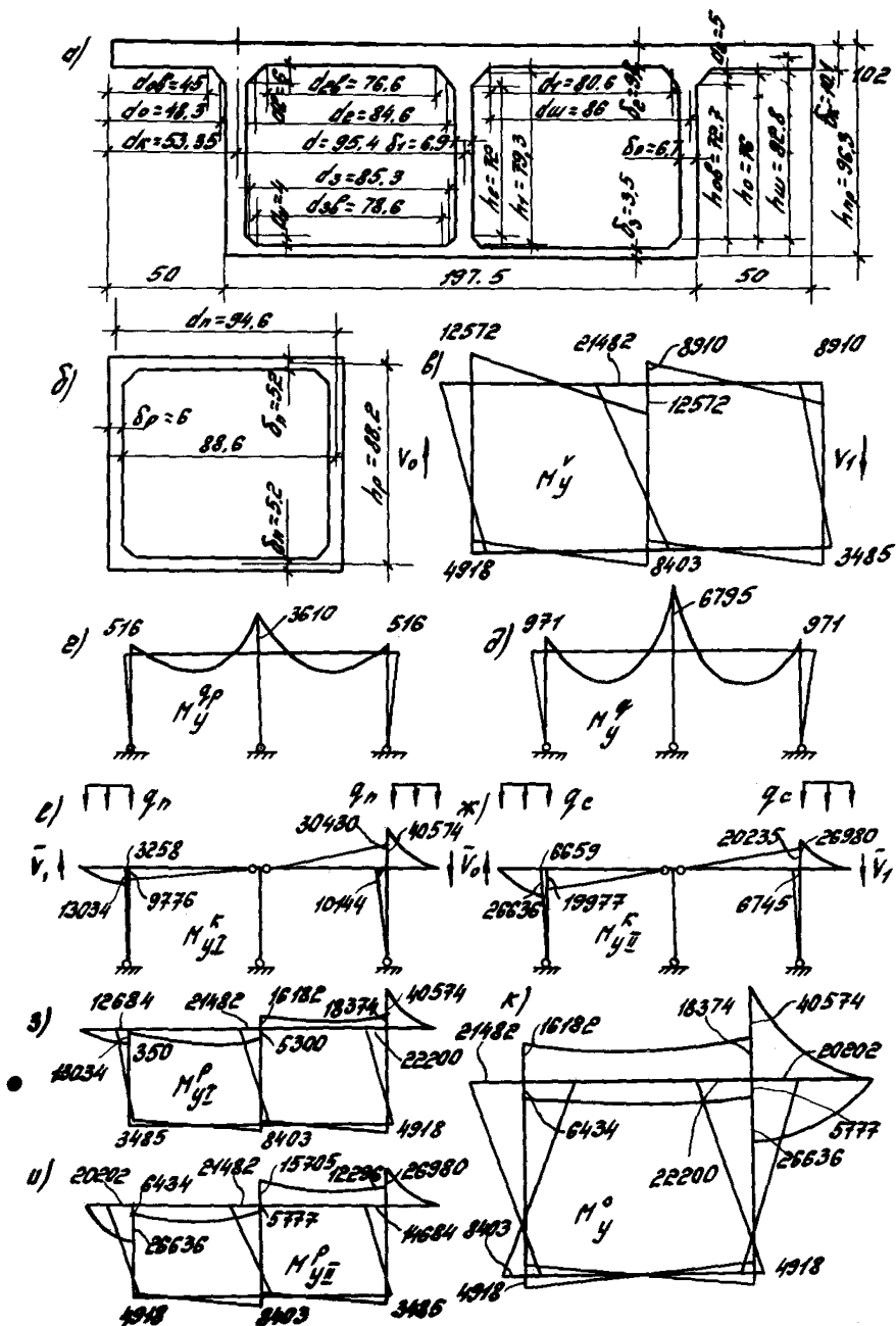
Рис. 4. Пример пространственного расчета коробчатого настила
