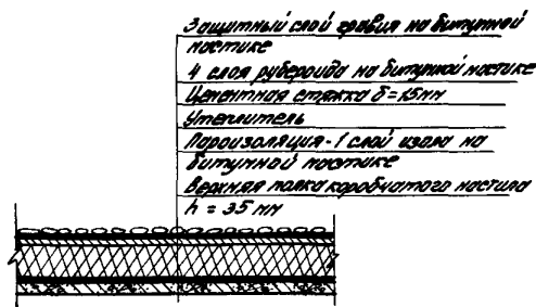
Рис. 26. Состав покрытия с корабчатыми настилами
