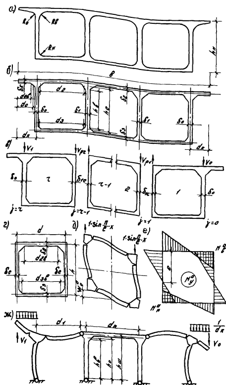
Рис. 2. Пространственный расчет коробчатого настила перекрытия
