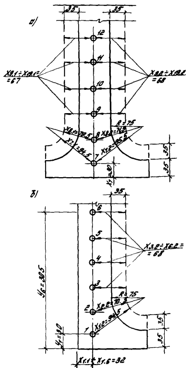
Рис. 24. Расчетная схема огневого воздействия на коробчатый настил номиналь- ной длины 18,0 м
