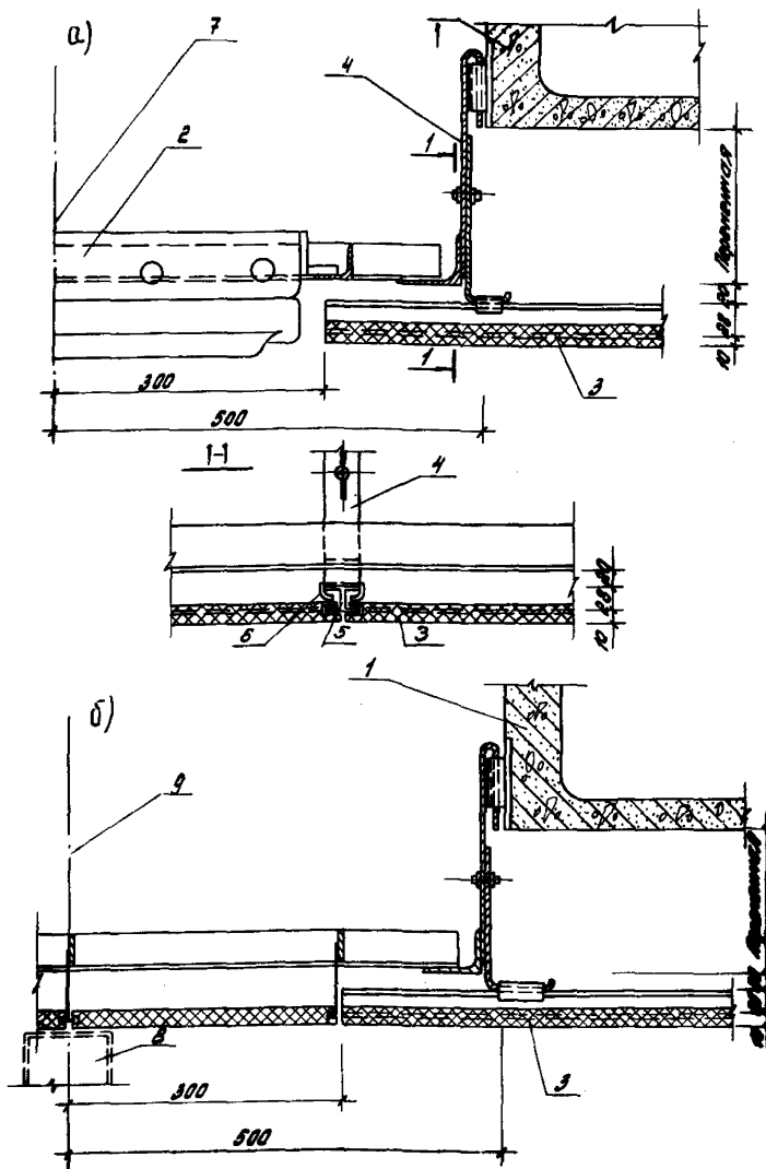
Рис. 8. Схема установки встроенных (а) и подвесных (б) светильников и устройства акустических потолков с относом от коробчатых настилов
