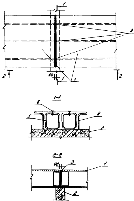
Рис. 7. Схема жесткой заделки узлов сопряжений торцов коробчатых настилов
