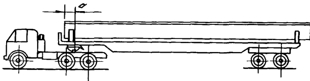
Рис. 17. Общий вид автопоезда с коробчатым настилом в транспортном положении
