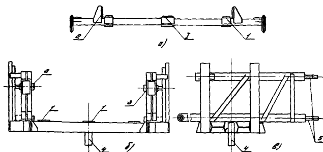
Рис. 15. Схемы промежуточной (а) и поворотной (б,в) рам
