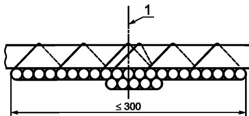
Рисунок 2 — Кабели, закрепленные на передней стороне стандартной лестницы без зазора (комплекты отрезков кабелей находятся в контакте)
