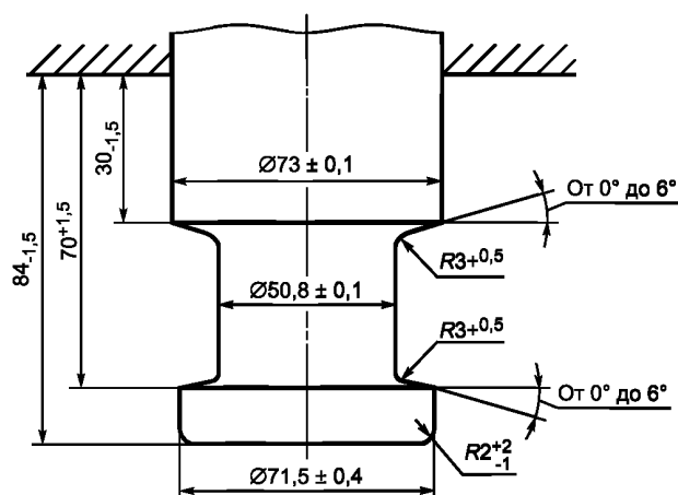
Рисунок 18 — Размеры шкворней седельно-сцепных устройств класса Н50
