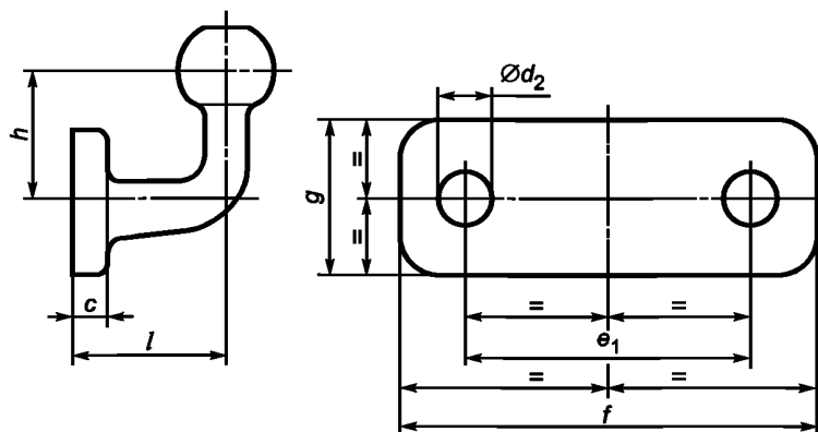
Рисунок 3 — Размеры стандартных фланцевых шаровых наконечников класса A50-1 (см. таблицу 6.1)
