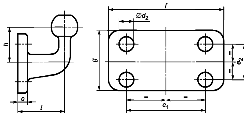
Рисунок 4 — Размеры стандартных фланцевых шаровых наконечников классов A50-2 — A50-5 (см. таблицу 6.1)
