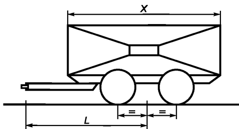
Рисунок 1 — Габаритные размеры прицепа с центрально расположенной осью
