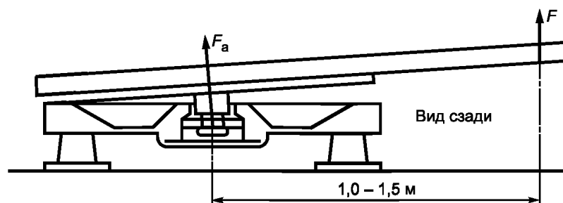
Рисунок 24 — Испытание седельно-сцепных устройств на подъем
