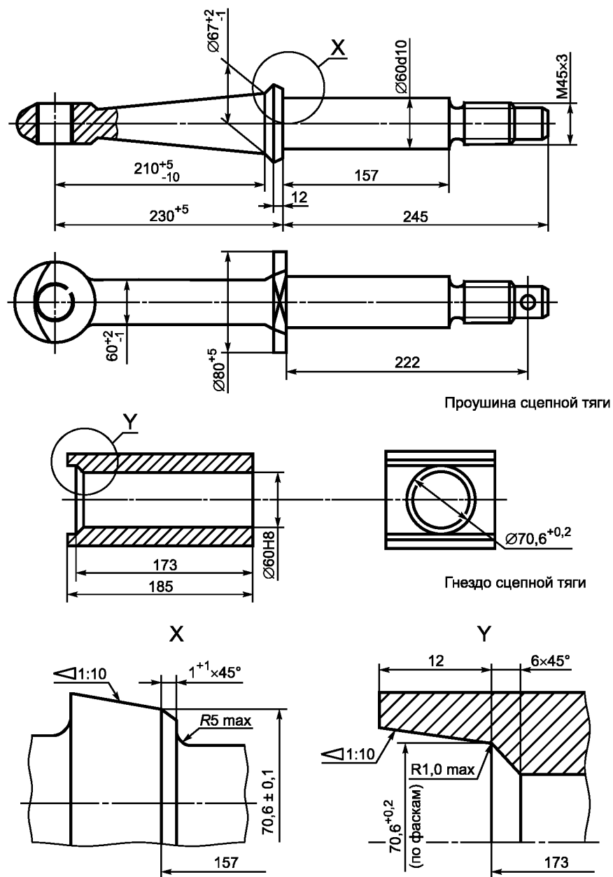
Рисунок 12 — Размеры проушин сцепных тяг класса D50-B
