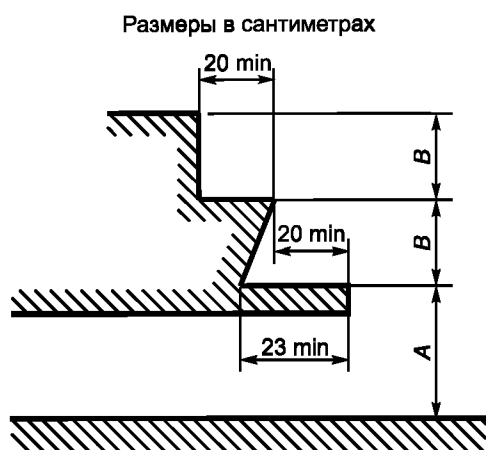
Рисунок 4 — Ступеньки у служебных дверей (см. 5.7.7)
