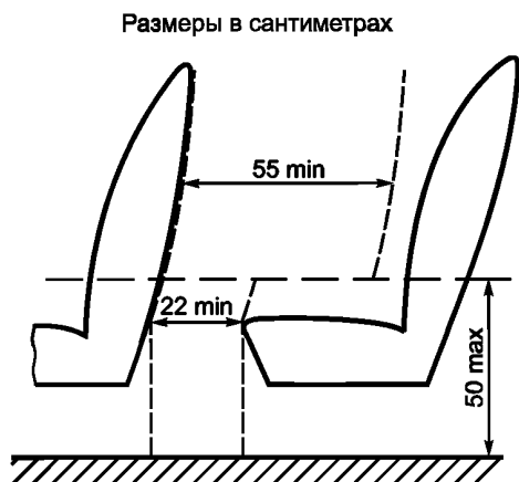
Рисунок 19 — Определение свободного доступа к двери (см. 5.7.1.10.1)
