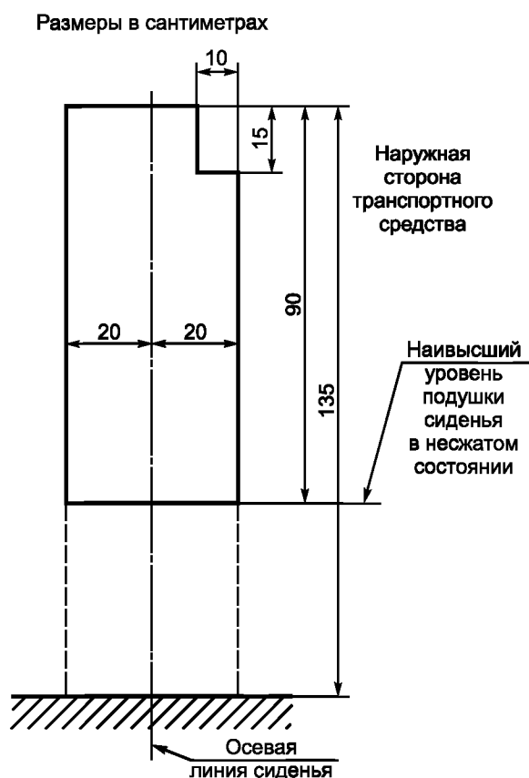
Рисунок 6 — Допустимое выступание конструкции внутрь зоны над сиденьем. Поперечное сечение минимально свободного пространства над сиденьем, размещенным возле боковой стенки транспортного средства (см. 5.7.8.1.2)
