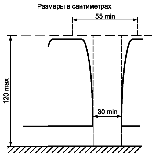
Рисунок 20 — Определение свободного доступа к двери (см. 5.7.1.10.2)
