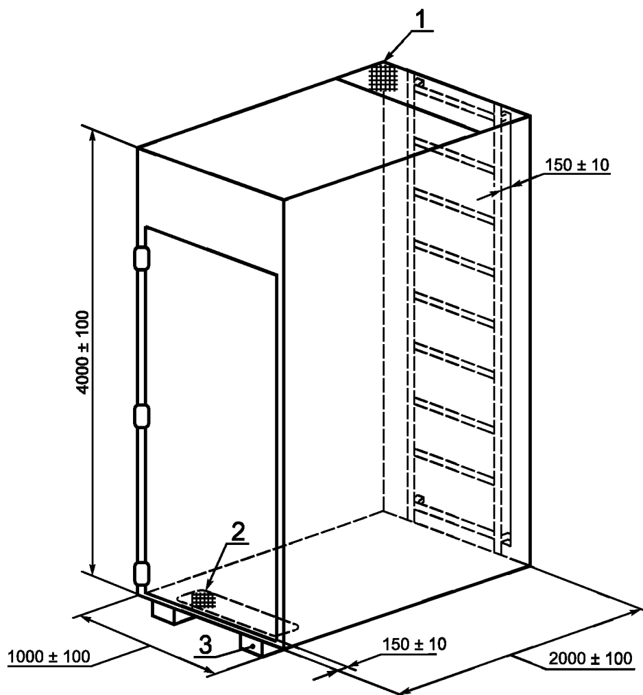
Рисунок 1 — Испытательная камера
