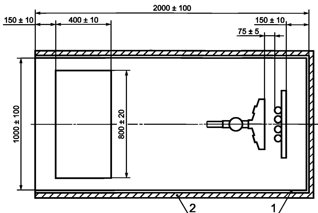
1 — стальной лист толщиной 1,5—2,0 мм; 2 — термоизоляция из минеральной ваты толщиной приблизительно 65 мм с соответствующим внешним покрытием, обеспечивающим коэффициент теплопередачи около 0,7 \text{ Вт} \cdot \text{м}^{-2} \cdot \text{К}^{-1}
