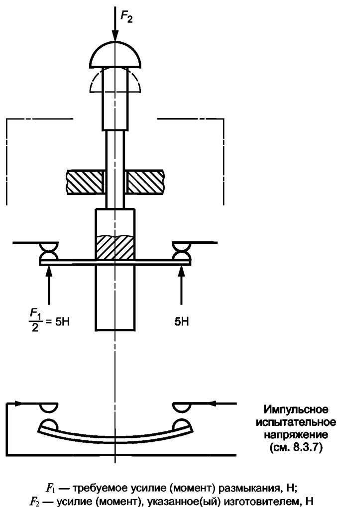
Рисунок К.1 — Проверка прочности механизма передачи усилия
