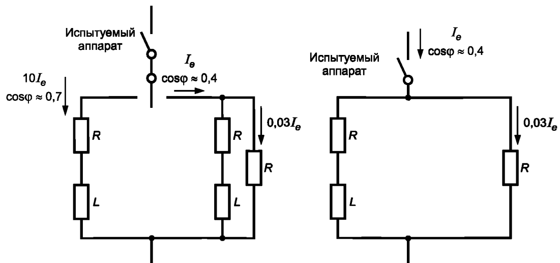
Рисунок С.1 — Полная схема (см. С.3.2.1)
