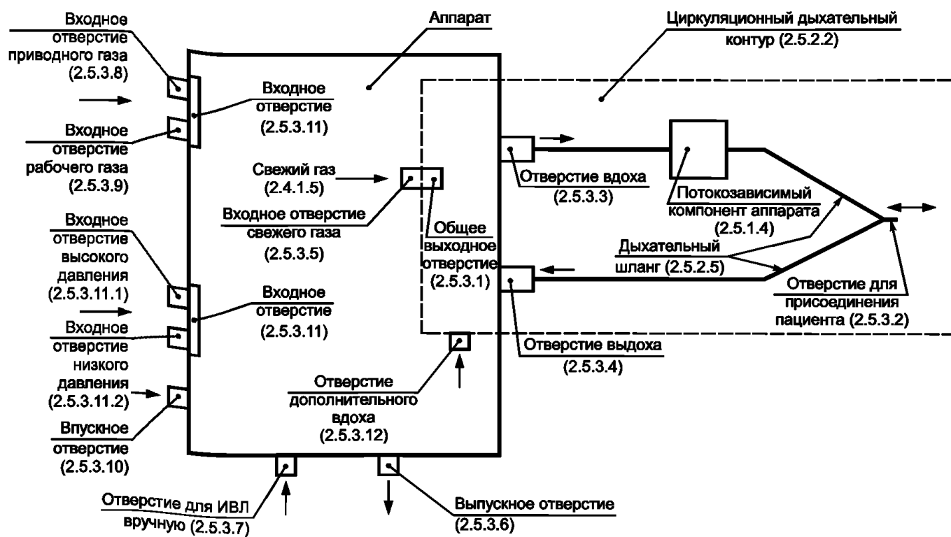
Рисунок А.1 — Схема расположения отверстий
