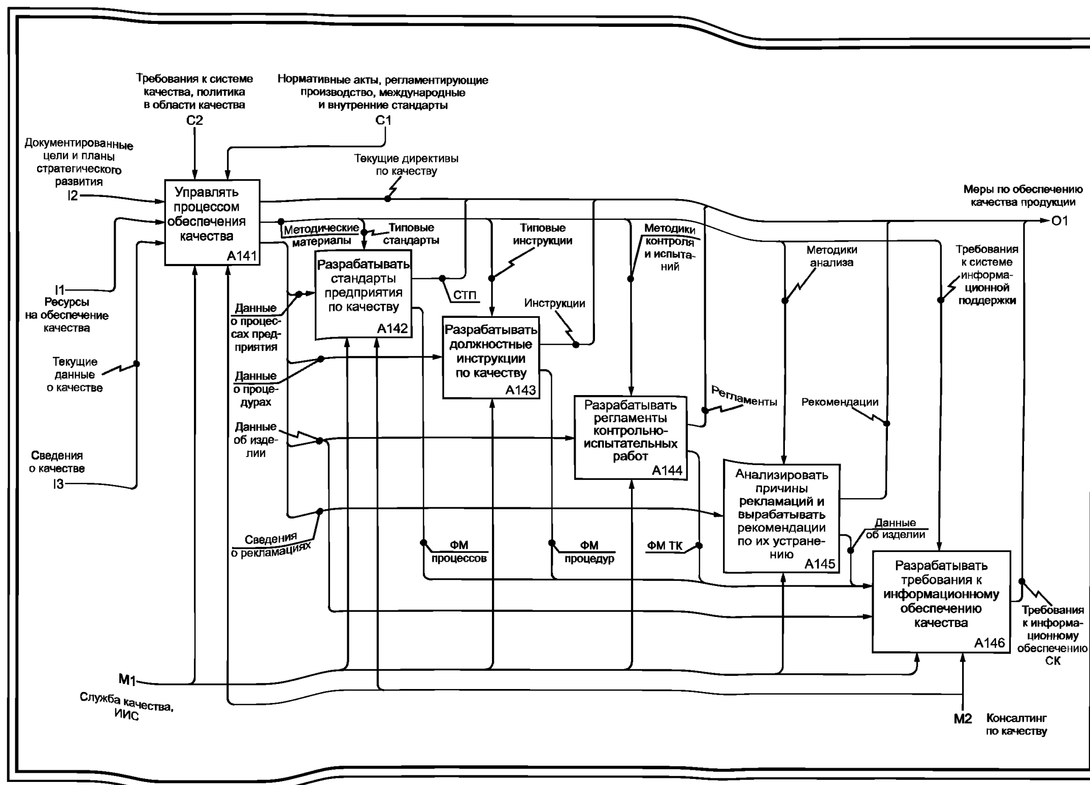
Рисунок В.4 — Декомпозиция блока А14
