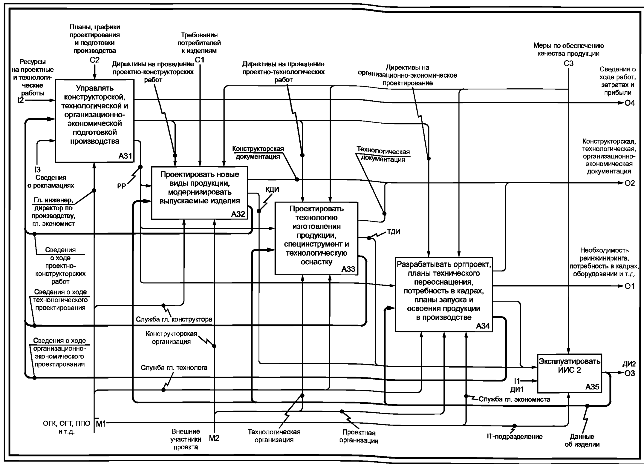
Рисунок В.5 — Декомпозиция блока А3
