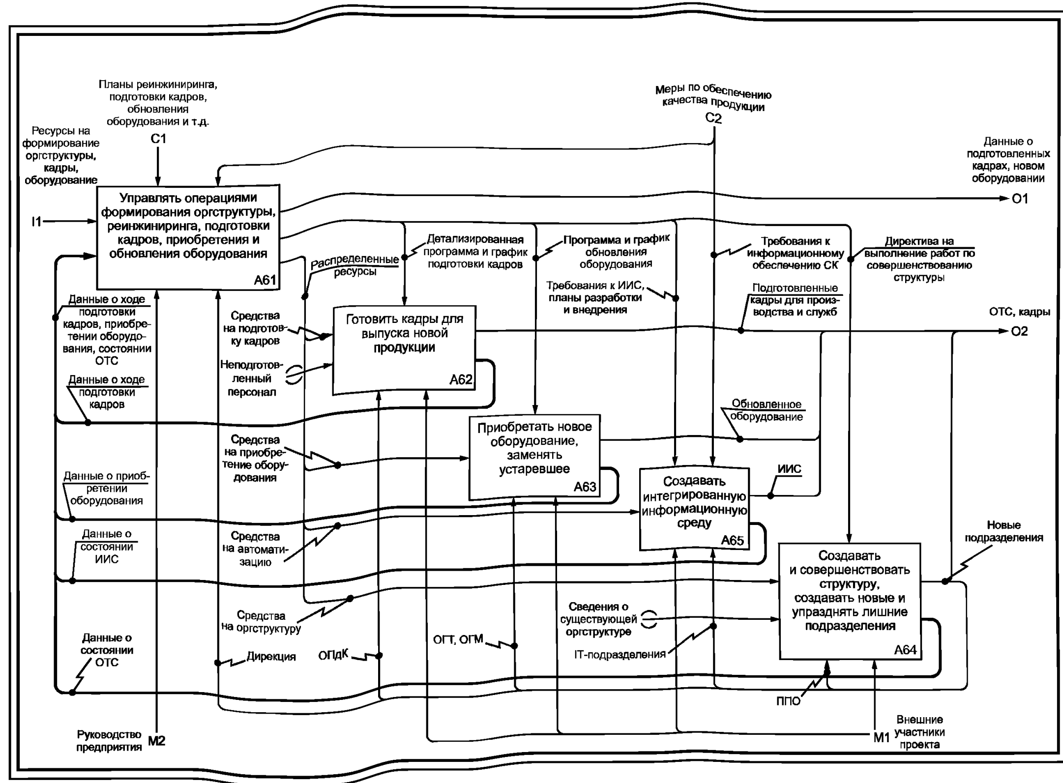
Рисунок В.7 — Декомпозиция блока А6
