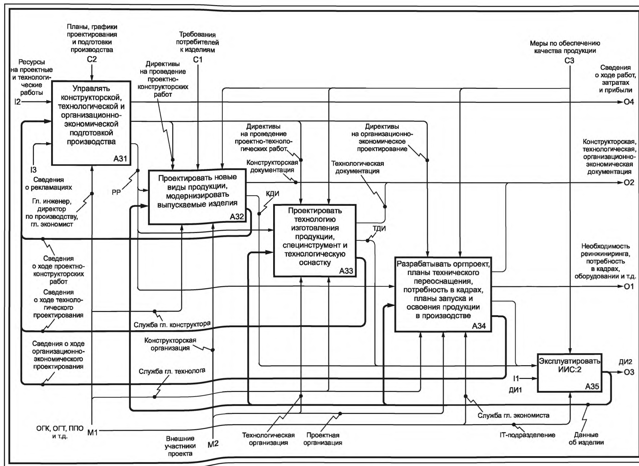
Рисунок Б.5 — Декомпозиция блока А3
