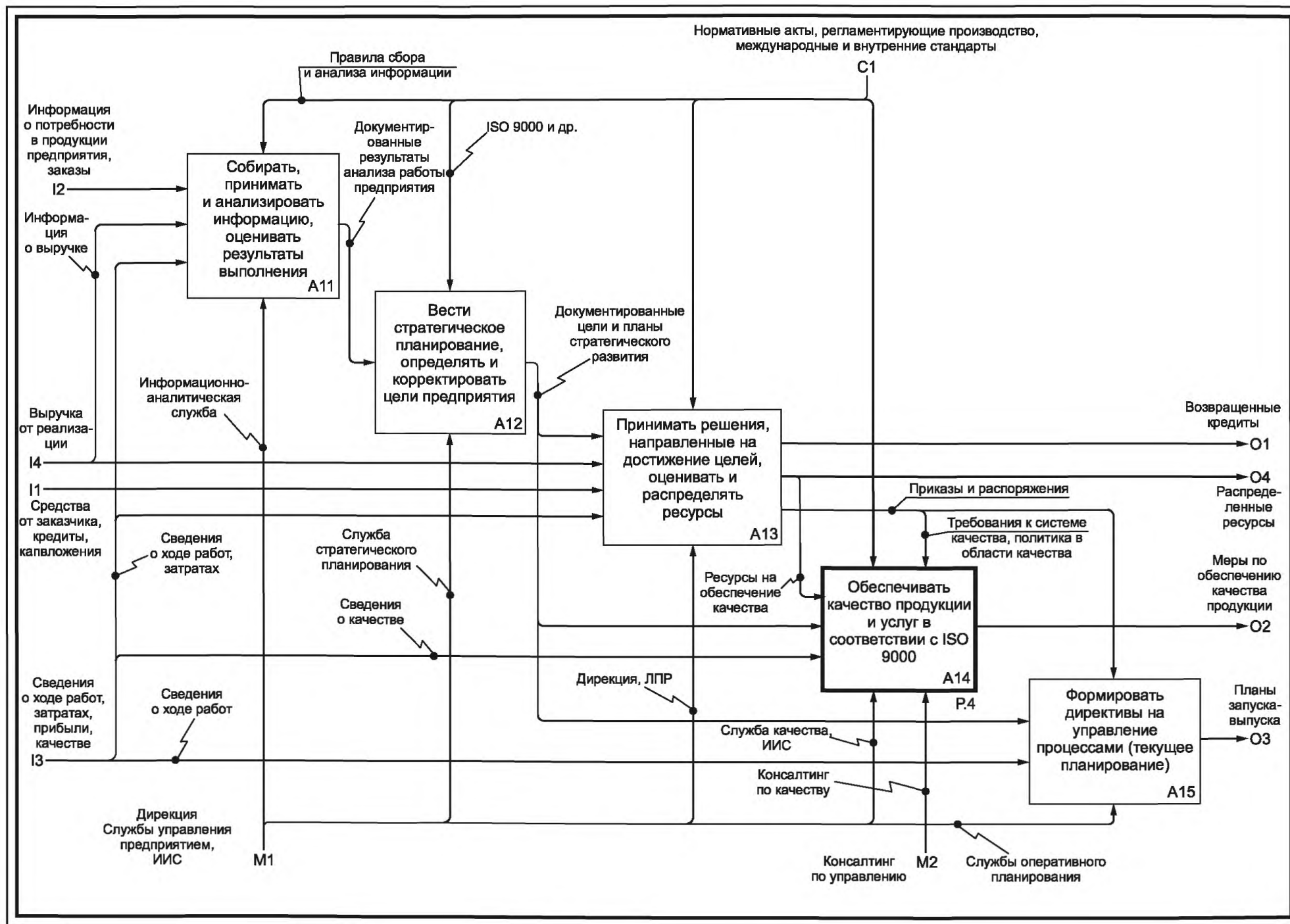
Рисунок В.3 — Декомпозиция блока А1
