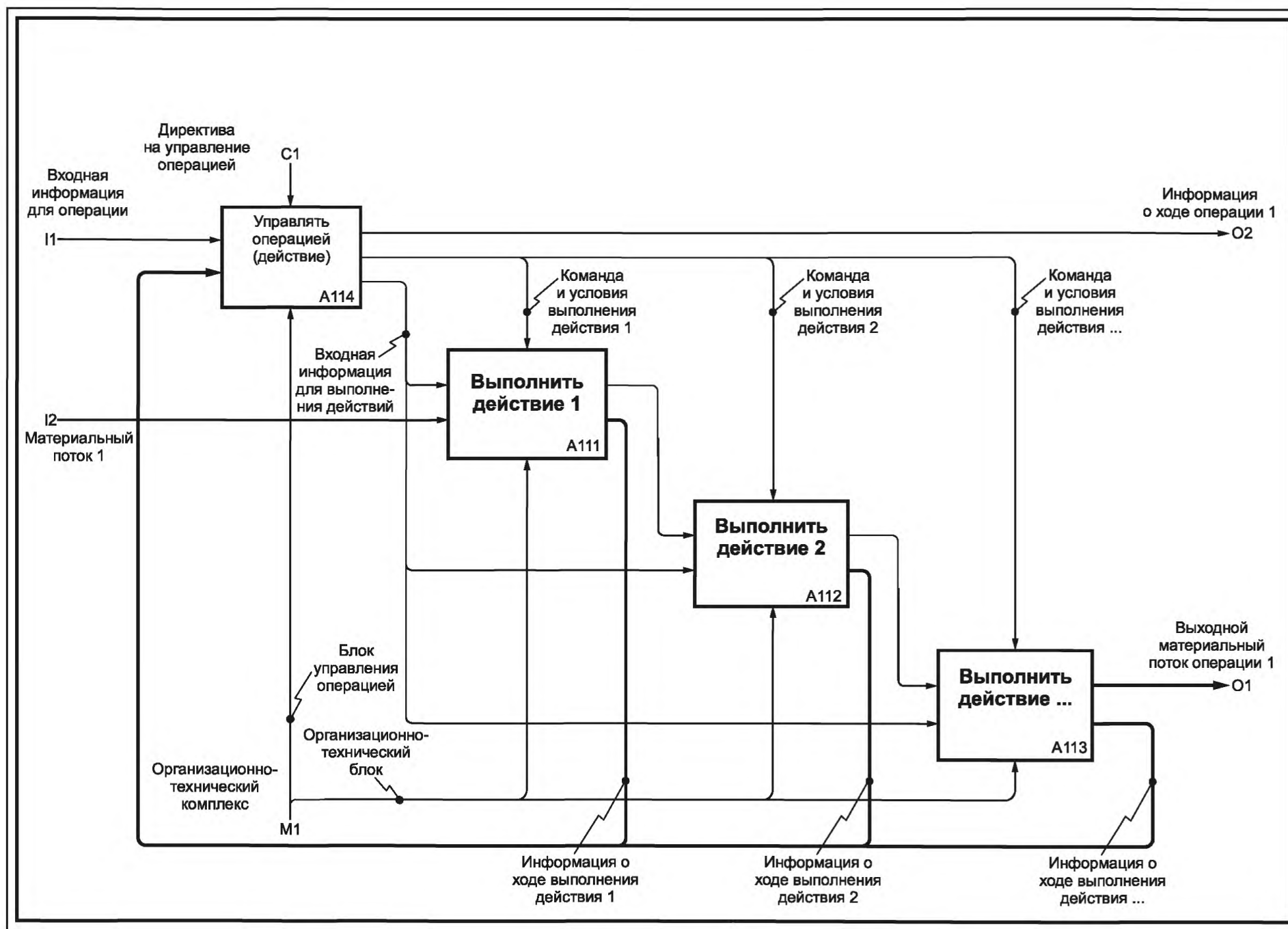
Рисунок Б.4 — Декомпозиция блока A11
