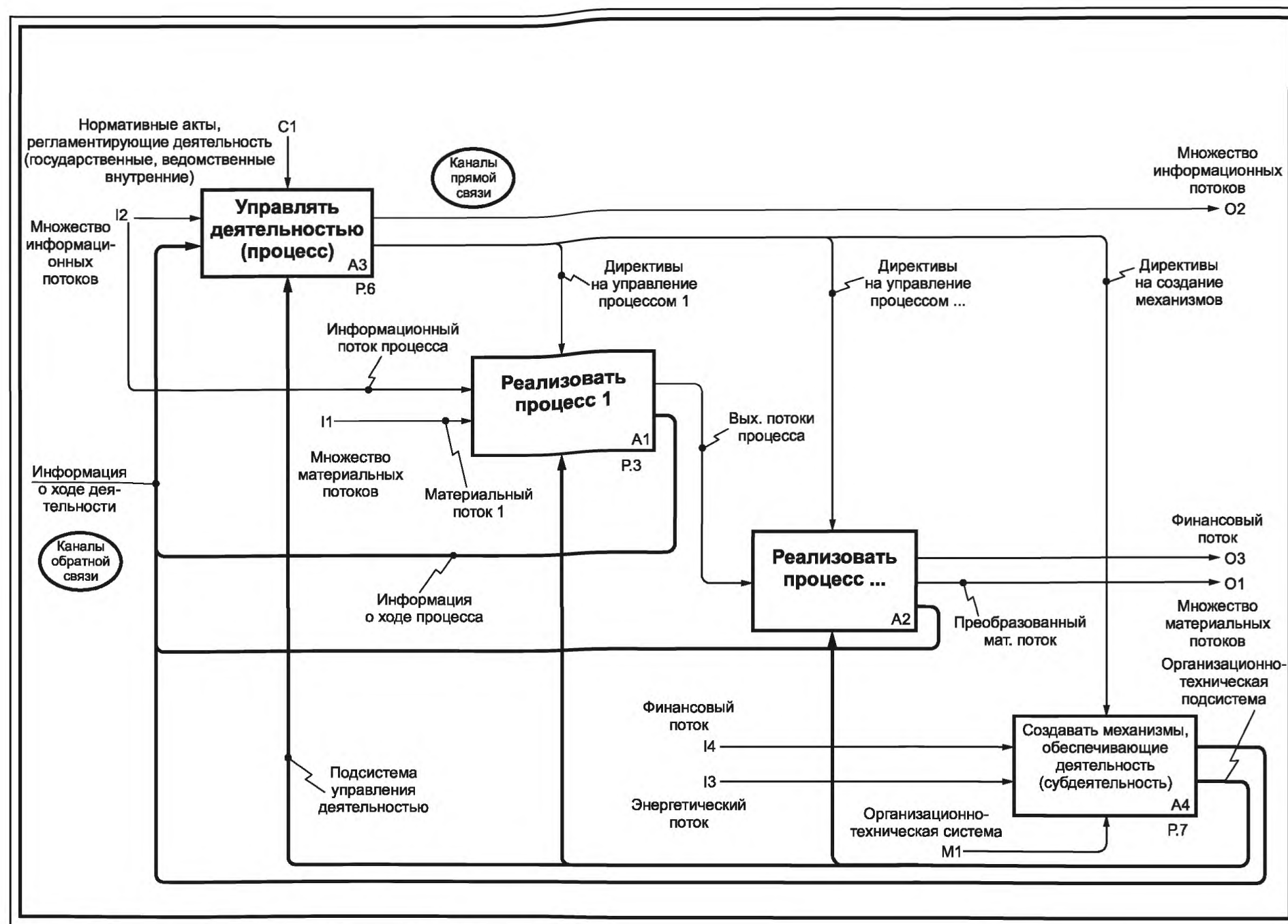
Рисунок Б.2 — Декомпозиция контекстной диаграммы
