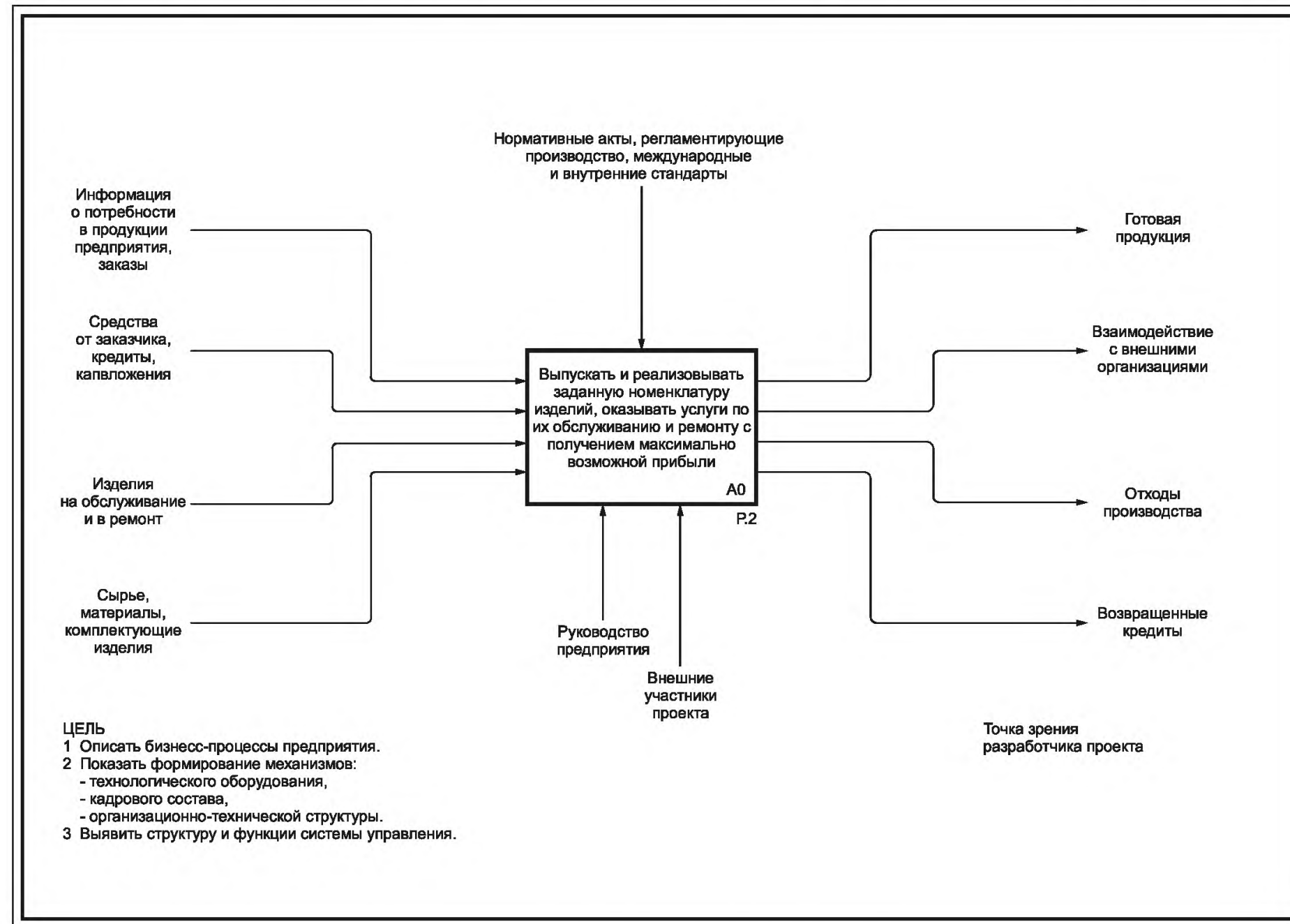
Рисунок В.1 — Контекстная диаграмма
