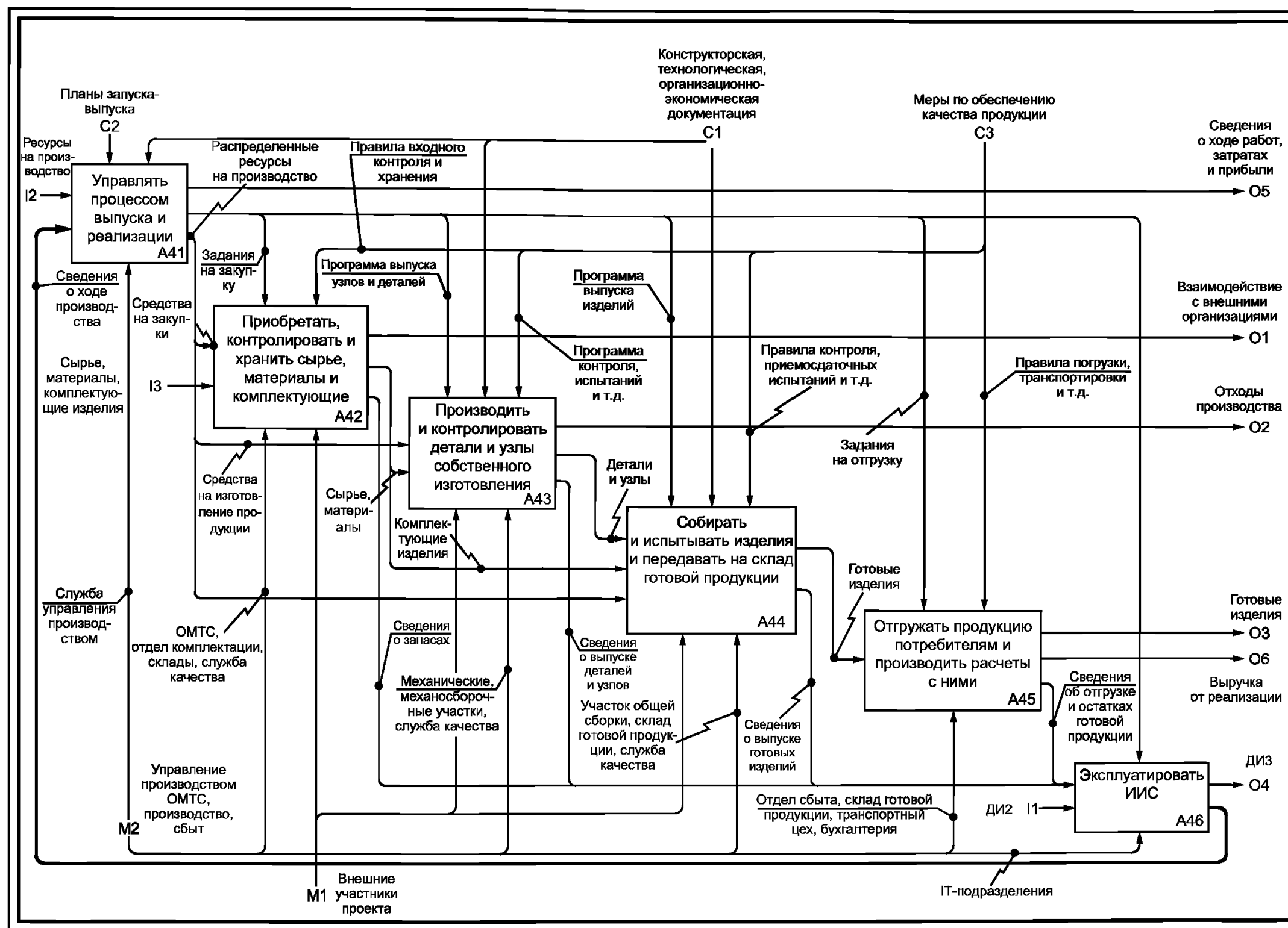
Рисунок В.6 — Декомпозиция блока А4
