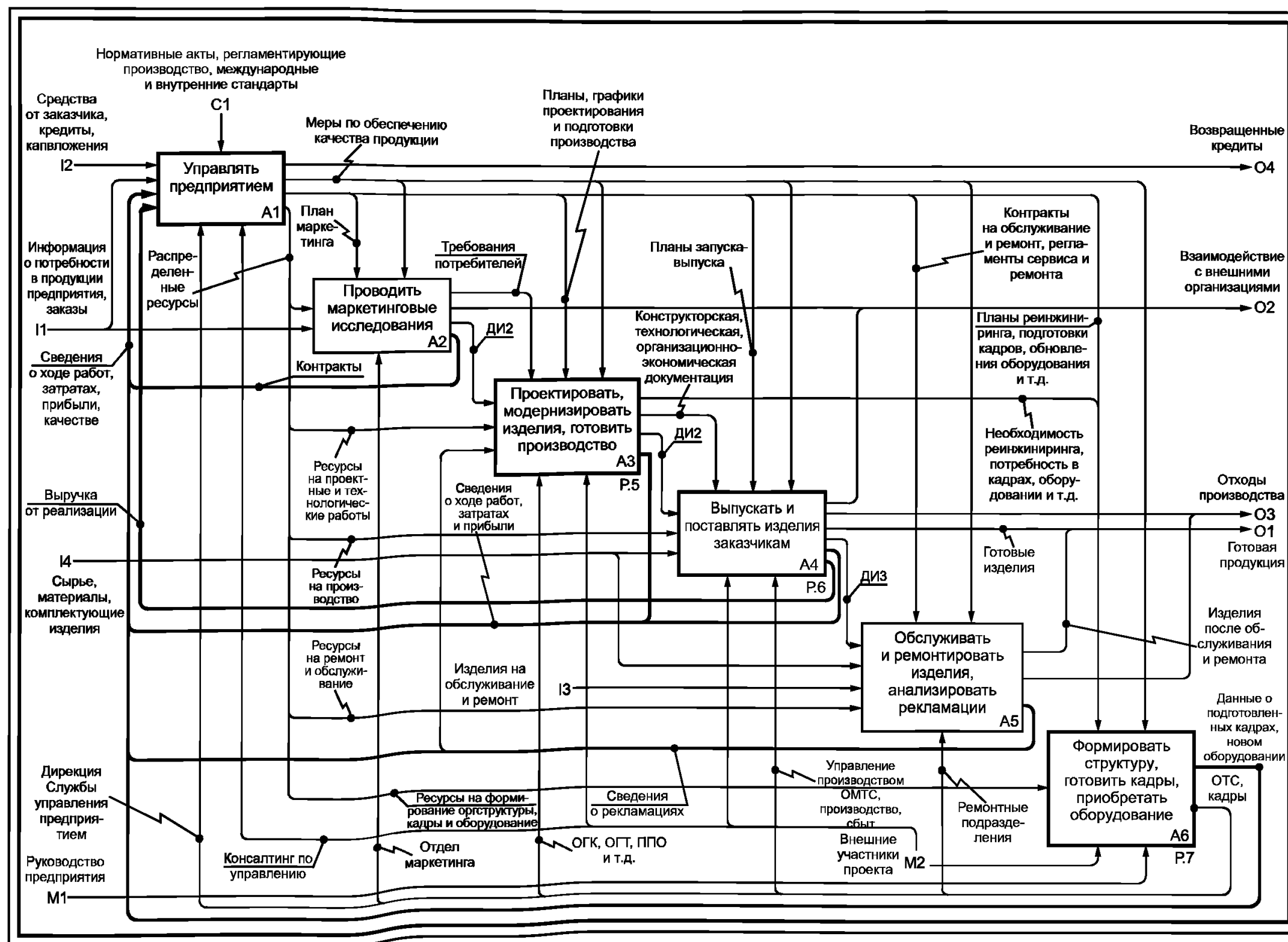
Рисунок В.2 — Декомпозиция контекстной диаграммы
