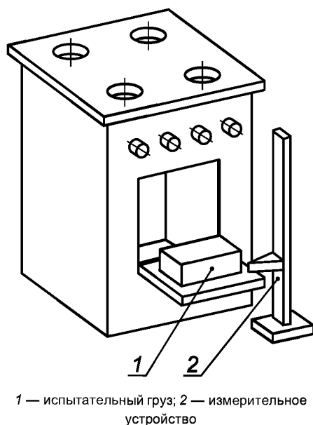
Рисунок 7 — Испытание на прочность дверцы духовки
