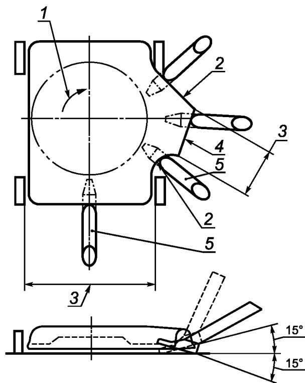
1 — направление вращения; 2 — сторона разгрузочного желоба, которую проверяют имитатором, если она менее чем на 3 мм ниже плоскости траектории движения лезвия режущего инструмента; 3 — область, проверяемая имитатором; 4 — разгрузочный проем; 5 — имитатор стопы (или основание имитатора из любого указанного начального положения)
