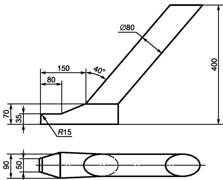
Рисунок 103 — Имитатор стопы
