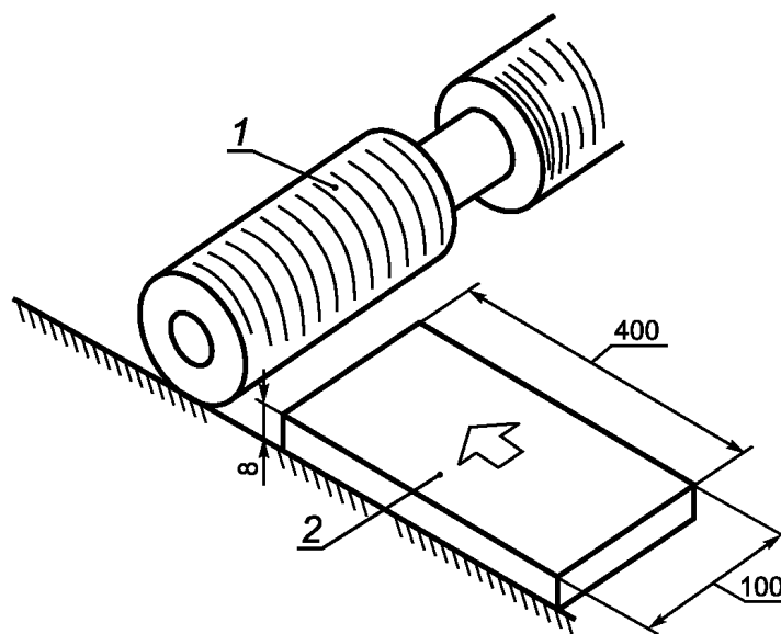
1 — режущее устройство; 2 — стальная пластина
