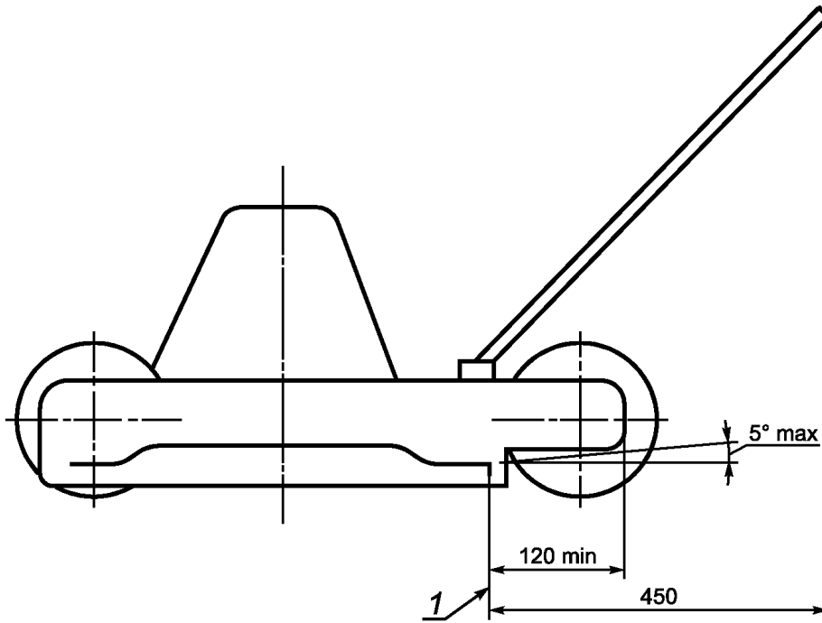
Рисунок 101 — Безопасные расстояния для ротационных приборов
