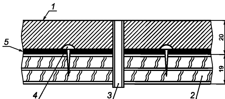
1 — кокосовый мат (квадрат размером 500 × 500 мм); 2 — основание из фанеры; 3 — труба подачи; 4 — гвоздь; 5 — поливинилхлоридное основание
