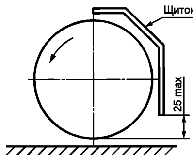
Рисунок 110 — Ограждение передних разгрузочных проемов
