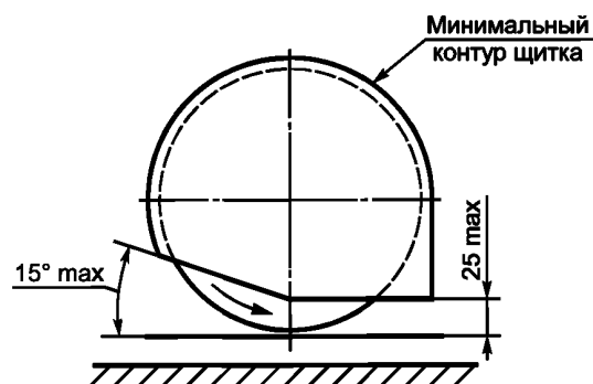
Рисунок 108 — Ограждение режущих устройств сбоку
