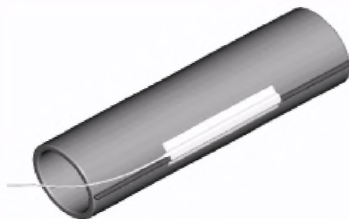
Рисунок 8 — Датчик ограничивающего устройства на поверхности электронагревателя
