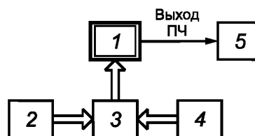
Рисунок 11 — Схема подключения оборудования при определении значений точек пересечения по интермодуляции второго IP_2 и третьего IP_3 порядков
