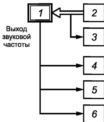
Рисунок 10 — Схема подключения оборудования при определении чувствительности приемника
