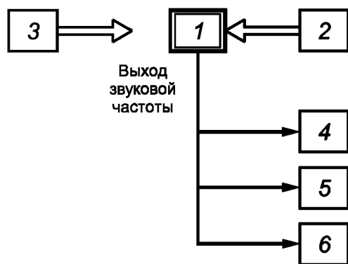
Рисунок 9 — Схема подключения оборудования при проверке ослабления помехи промежуточной частоты, сигналов зеркальных частот и помех по побочным каналам приема
