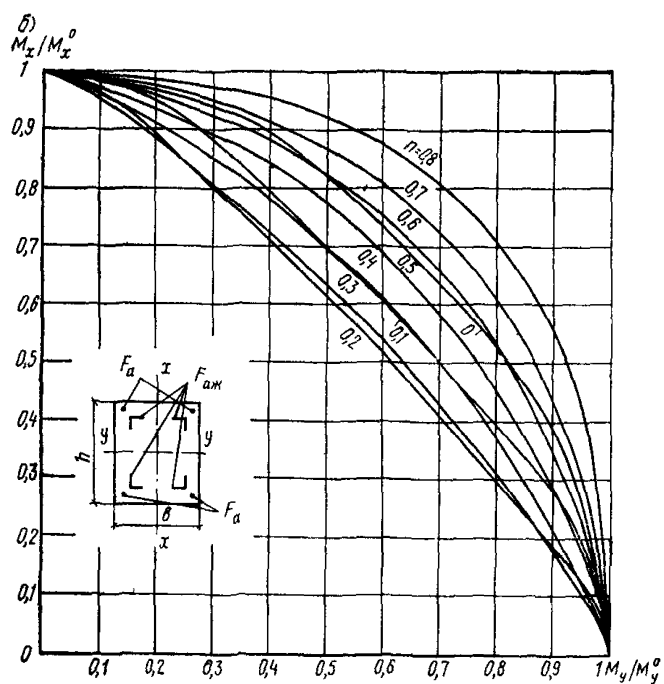
Рис. 16. График несущей способности прямоугольного сечения при косом внецентренном сжатии с жесткой арматурой а — в виде двутавра; б — в виде уголка
