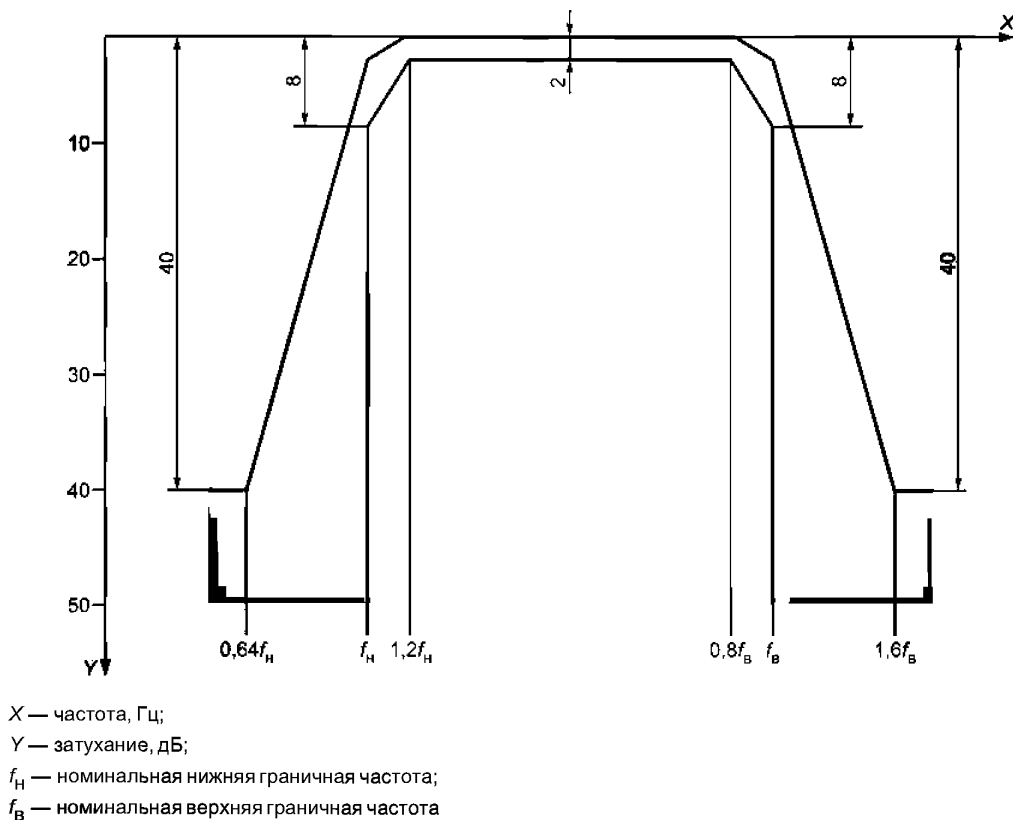
Рисунок 4 — Поле допуска АЧХ полосовых фильтров
