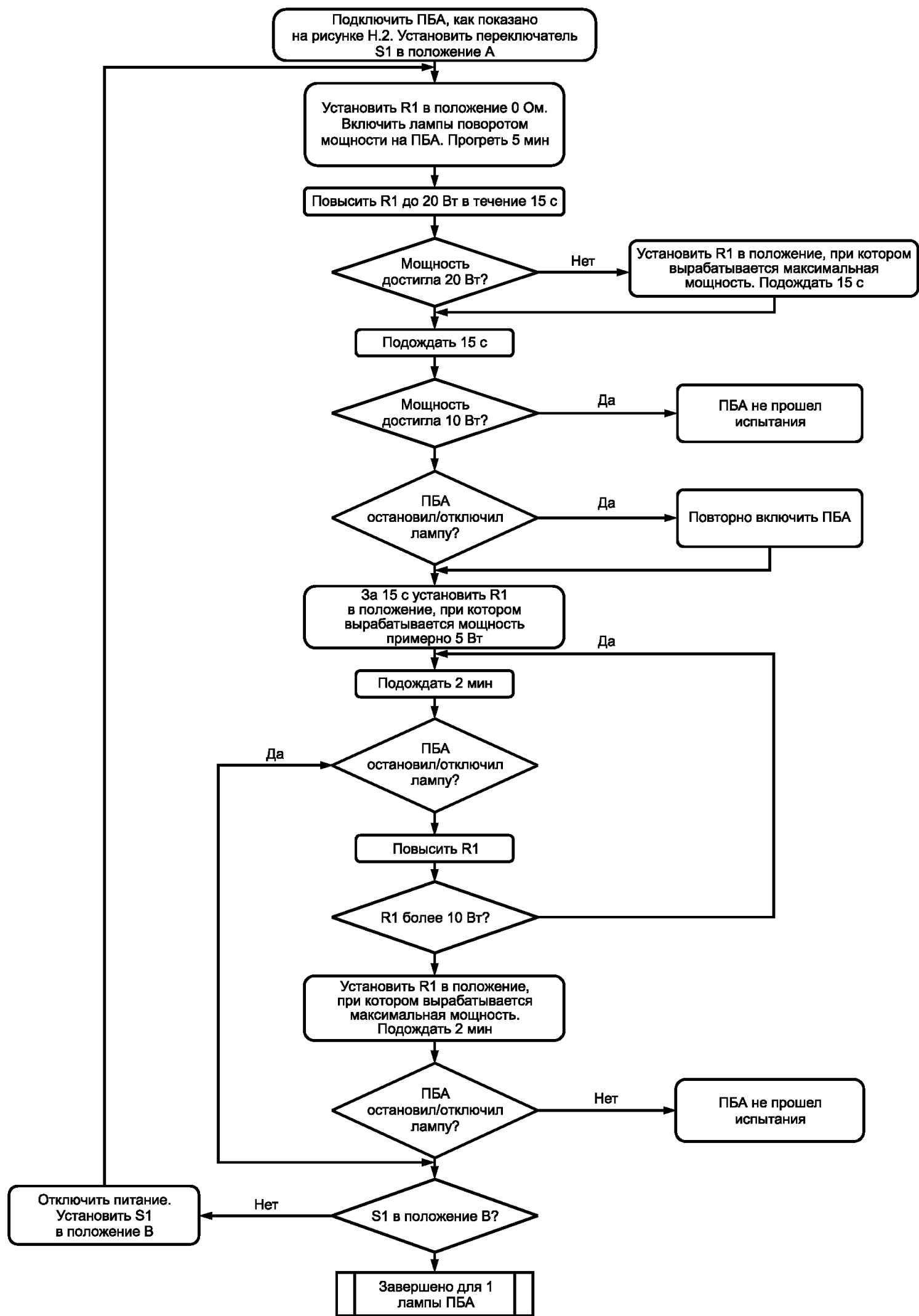
Рисунок Н.3 — Блок-схема испытания асимметричной мощностью
