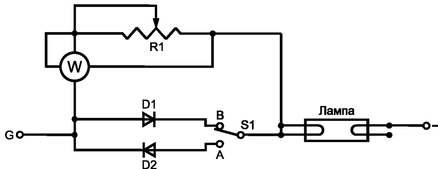
Рисунок Н.2 — Схема испытания асимметричной мощностью
