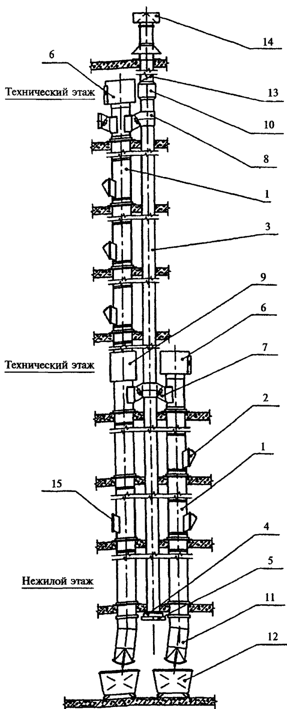
Рисунок 1. Система мусороудаления в высотных зданиях
