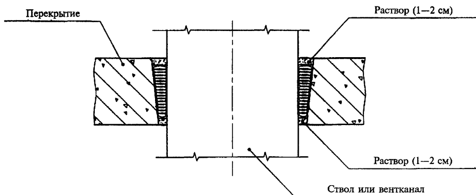
Рисунок 3. Звукоизоляция междуэтажных перекрытий
