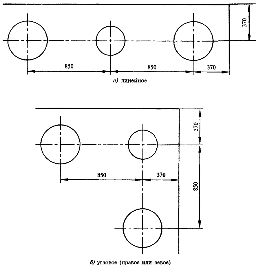
Рисунок 2. Взаимное расположение проемов в перекрытиях под ствол и вентканал
