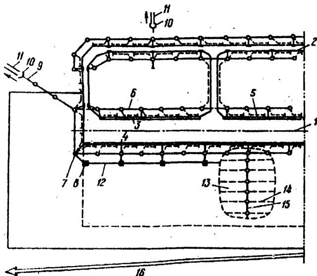
Рис. 5.1. Общий вид расположения водоотводных систем на аэродромах: 1 — ИВПП; 2 — РД; 3 — лоток; 4 — дождеприемник; 5 — закрываемые дренажи; 6 — коллектор; 7 — смотровой колодец; 8 — тальвежный колодец; 9 — главный коллектор; 10 — устье (оголовок); 11 — открытая водоотводная канава; 12 — ось грунтового лотка; 13 — выборочное осушение грунтовых участков; 14 — осушитель; 15 — собиратель; 16 — нагорная канава.
