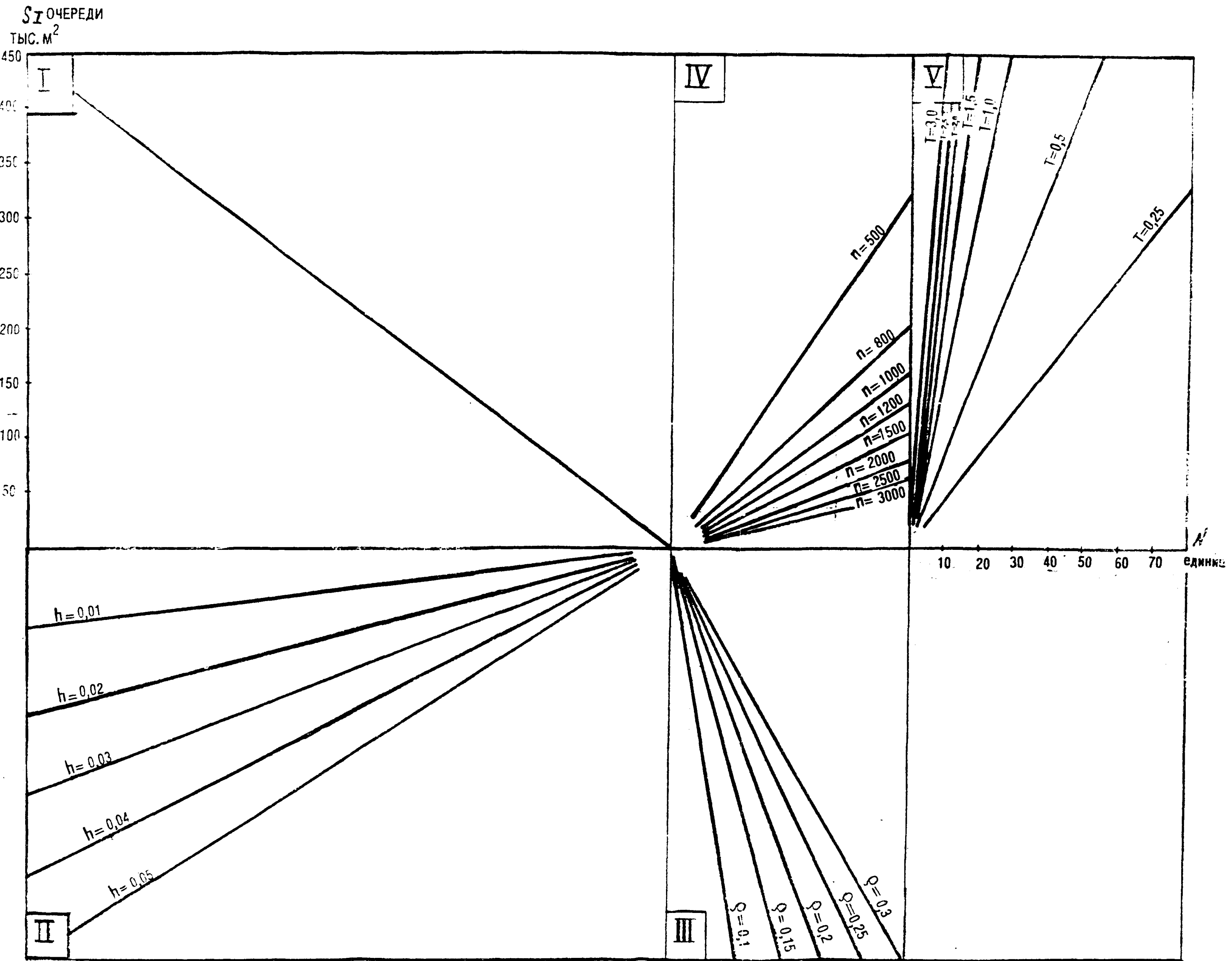
Рис. 2. Номограмма определения количества роторных снегоочистителей
