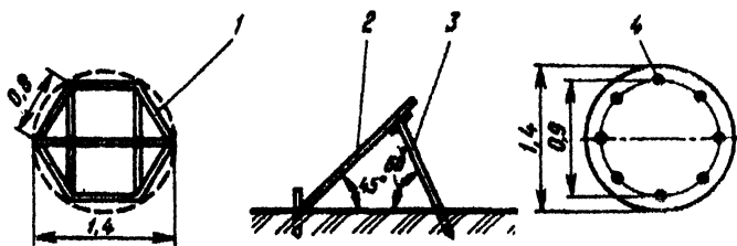
Рис. 3.13. Знак центра полосы:
