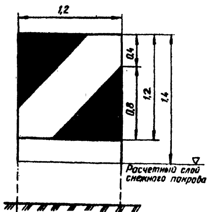
Рис. 3.18. Знак боковых границ.
