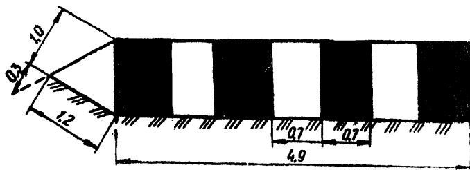
Рис. 3.17. Входной знак.
