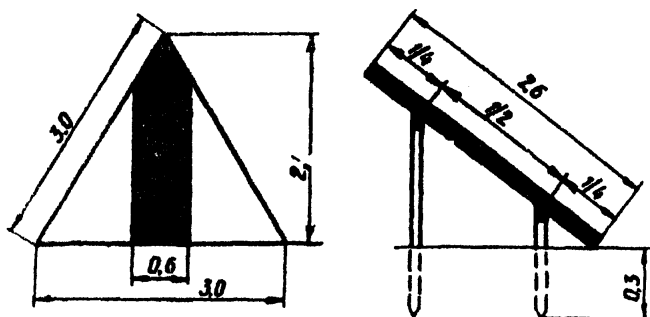
Рис. 3.20. Знак подхода.
