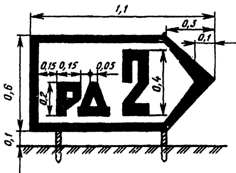
Рис. 3.21. Рулевой знак.
