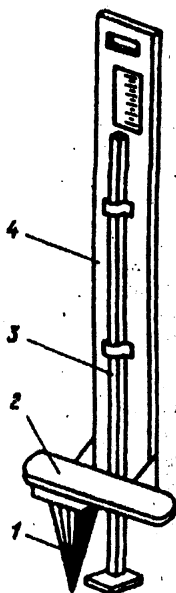
Рис. 1. Твердомер НИАС:
