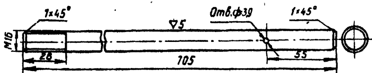
Рис. 4. Шток направляющий. Ст. 30ХГСА.
