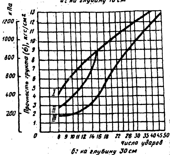
Рис. 5. Графики для определения прочности грунта ударником У-1: I — для песчаных, песчаных пылеватых, супесчаных и мелких супесчаных грунтов; II — для пылеватых, суглинистых, тяжелых суглинистых, суглинистых пылеватых и глинистых грунтов; III — для черноземов, каштановых и других засоленных грунтов.
