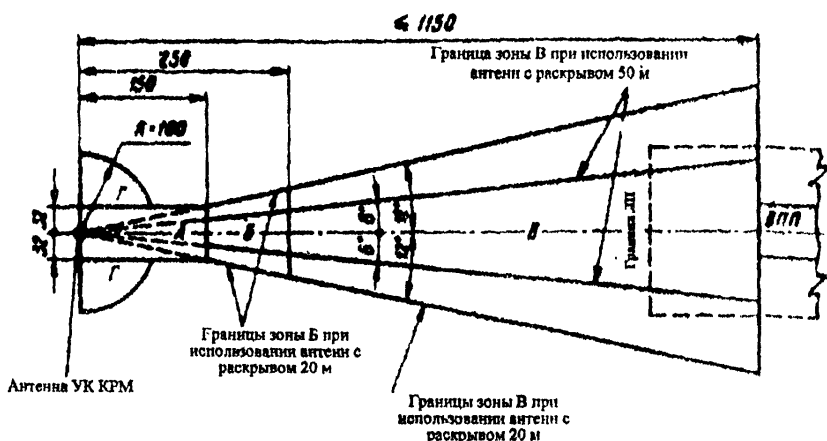
Рис. 2.2. Зоны КРМ РМС типа СII-70.
