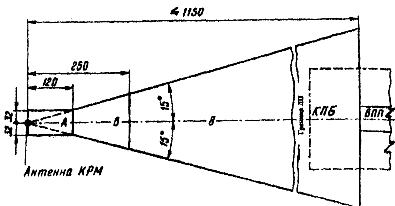
Рис. 2.1. Зоны курсового радиомаяка для РМС-1, СII-68.
