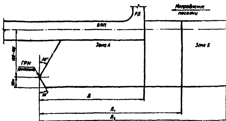
Рис. 2.5. Зоны глissадного радиомаяка СП-70, СП 80М.
