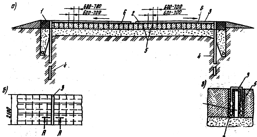
Рис. 5.3. Заземляющее устройство:
