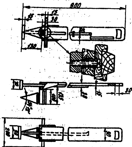
Рис. 2. Чертежи конусного твердомера.
