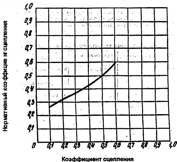
Рис. 3. Корреляционный график.
