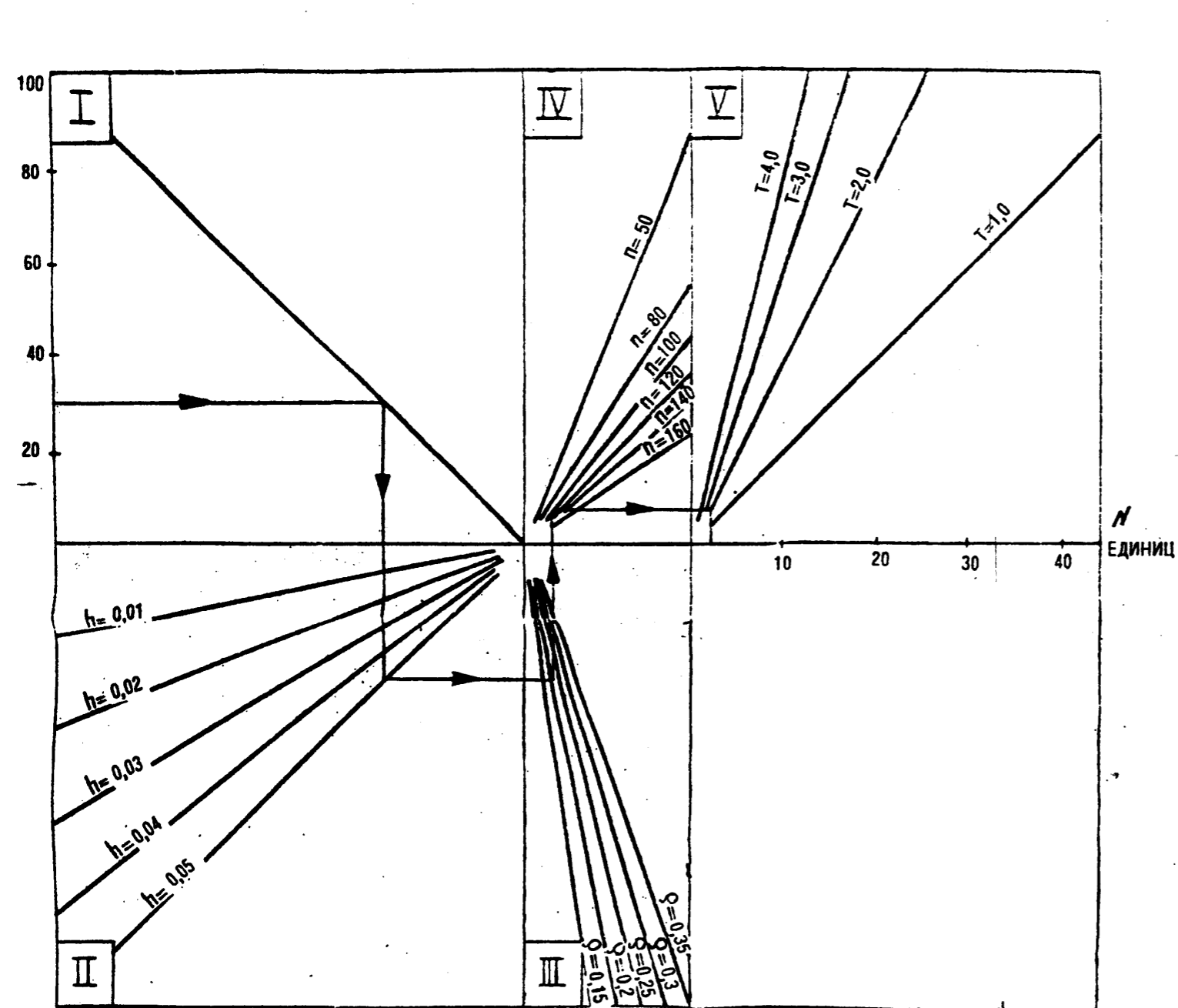
Рис. 3. Номограмма определения количества снегопогрузчиков
