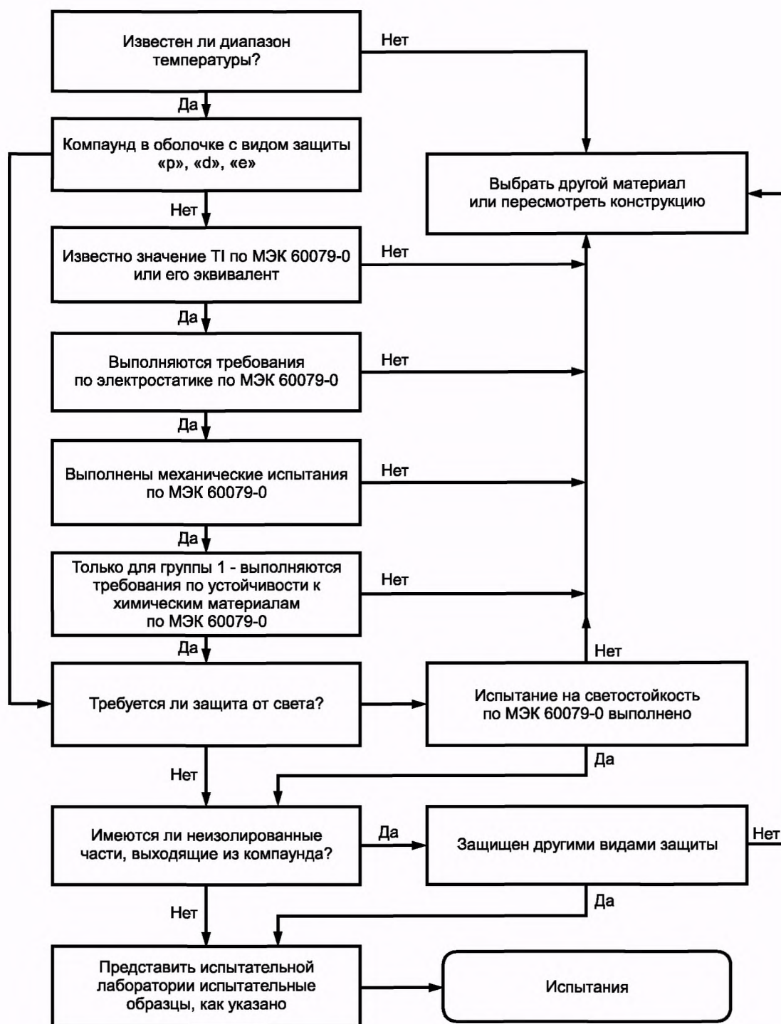
Рисунок А.1 — Основные требования к компаундам для оборудования с взрывозащитой вида «герметизация компаундом «т»
