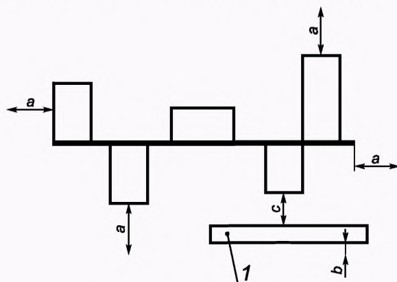
Рисунок 1 — Расстояния между наружной поверхностью компаунда и элементами или проводниками
