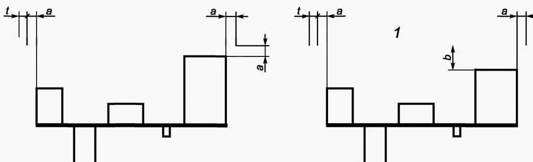
Пластмассовый корпус со всех сторон
