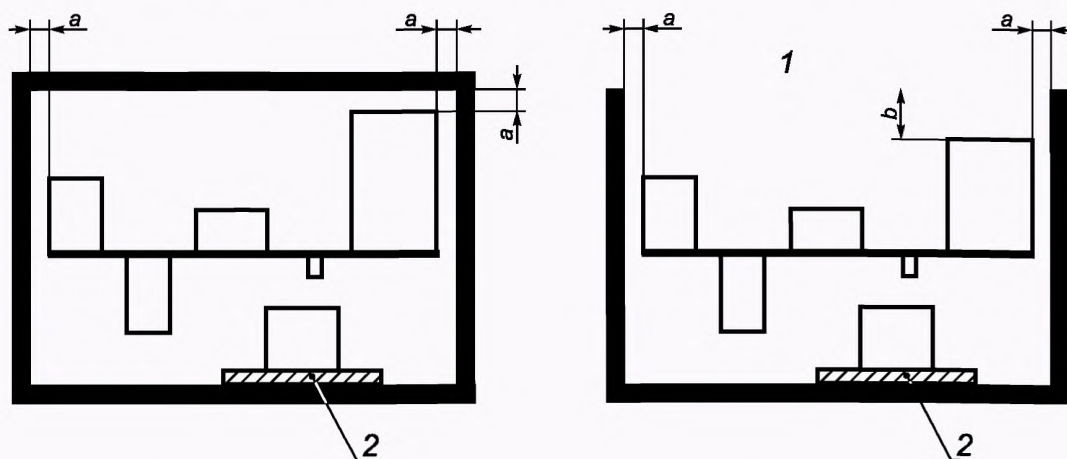
Рисунок 2 — Расстояния между стенкой или наружной поверхностью компаунда и элементами или проводниками
