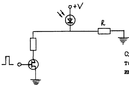
Транзисторная схема, используемая для аналоговой модуляции интенсивности излучения
