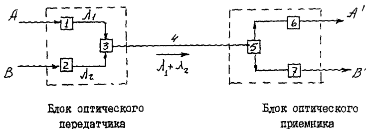
Схема мультиплексирования оптического сигнала
