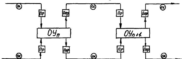
Пример активного подключения ОУ к сети с топологией системы магистраль или кольцо
