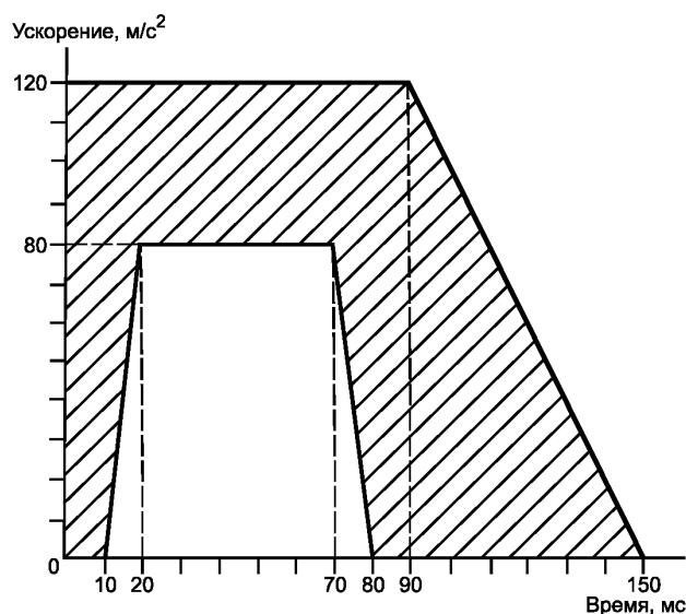
Рисунок 7.1 — Импульс ускорения
