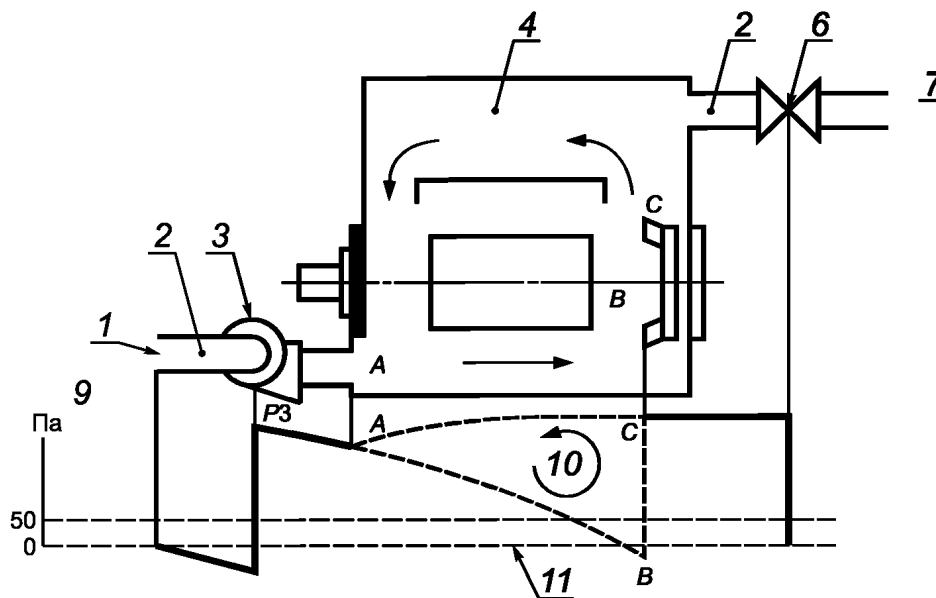
Рисунок С.2 — Оболочка под давлением с компенсацией утечки без подвижных частей
