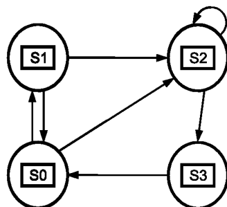
Рисунок В.1 — Диаграмма состояния системы управления продувкой с компенсацией утечки
