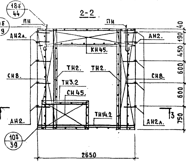
Арматурные блоки АНР5-28.26.3-45 и АНР5-28.26.3-48А.
