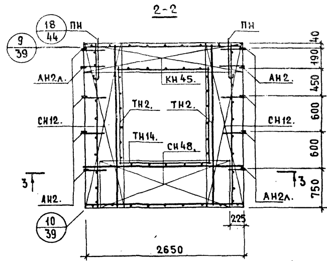
АРМАТУРНЫЙ БЛОК АНР5-28.29.3-3
