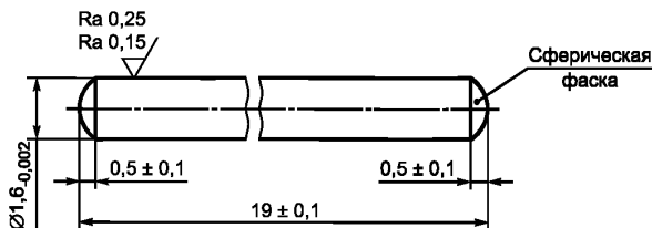
Рисунок 2 — Испытательный мандрен
