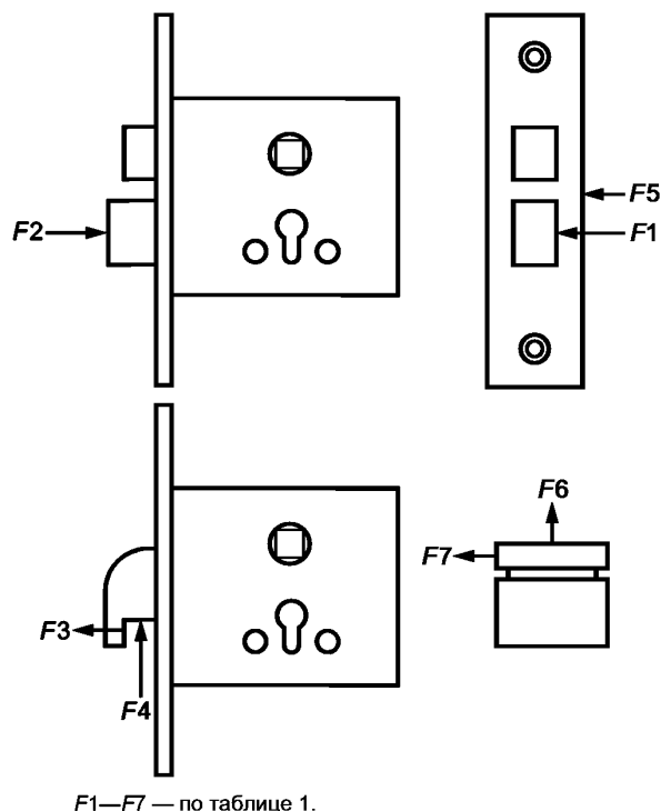
Рисунок 1 — Точки приложения сил, действующих на механизм замка
