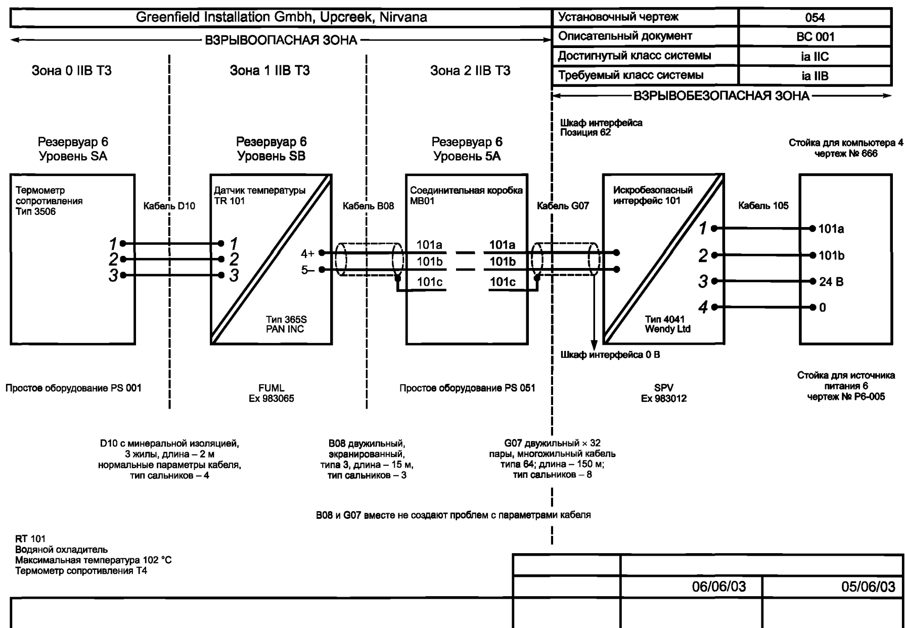
Рисунок E.2 — Типовой установочный чертеж для искробезопасной системы
