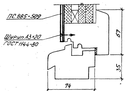
17-17 M1:2
