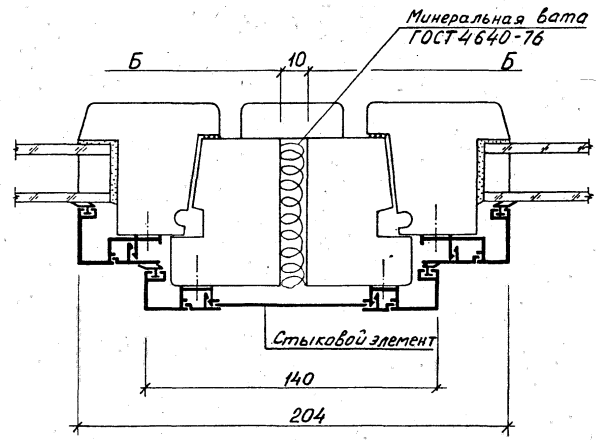
2-2 M 1:2
