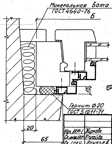
3-3 M 1:2
