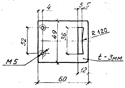
Деталь "Б"
