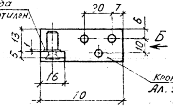
Деталь "А"
