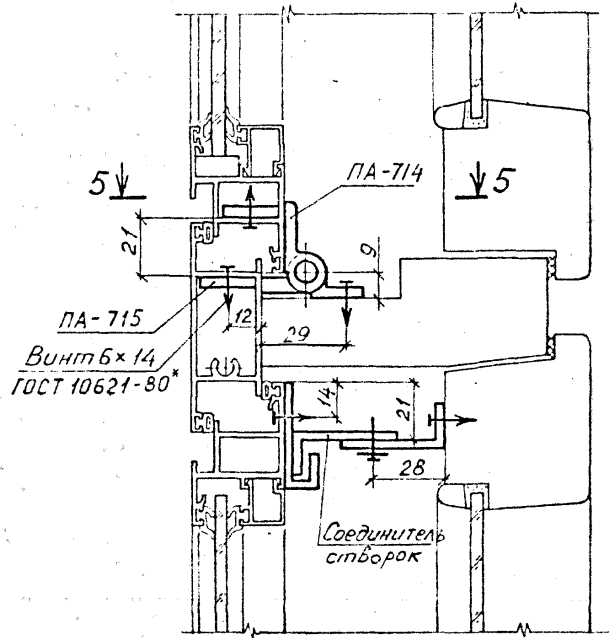
4-4 M 1:2
