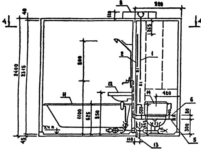
Рис 2 ДЕТАЛЬНОЕ - см. Рис. 1 1-1
