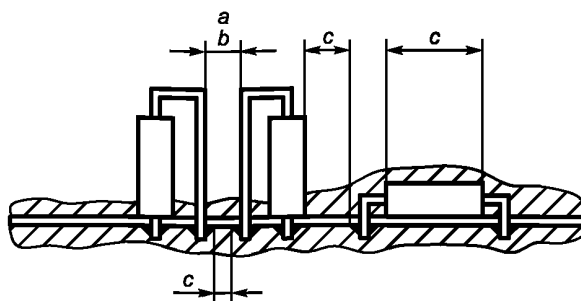
Рисунок c) — Плата с пайкой обрезанных или подогнутых выводов резисторов
