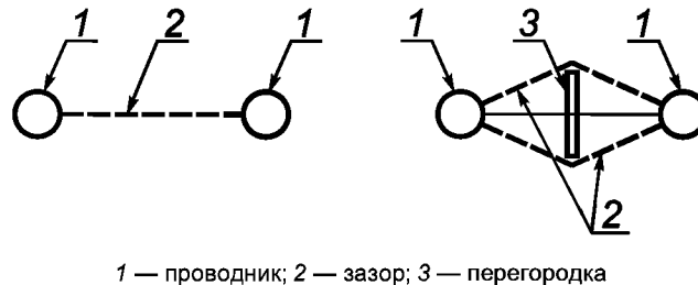
Рисунок С.1 — Измерение зазора
