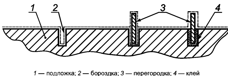
Рисунок С.3 — Измерение длины путей утечки
