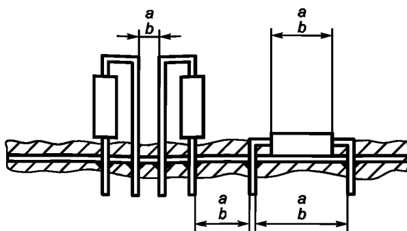
Рисунок b) — Плата с пайкой выступающих выводов резисторов
