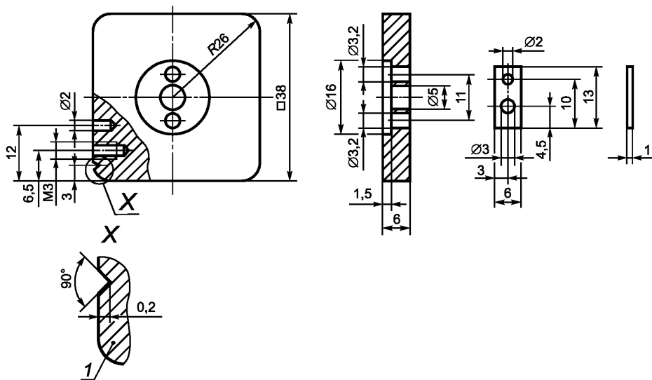
Рисунок В.3 — Держатель проволочек
