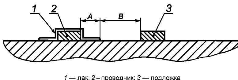
Рисунок С.4 — Измерение сложных расстояний
