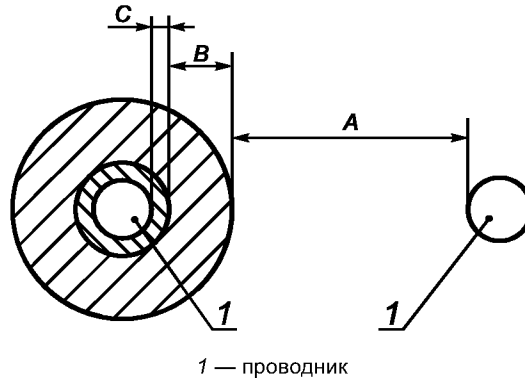
Рисунок С.2 — Измерение сложных расстояний
