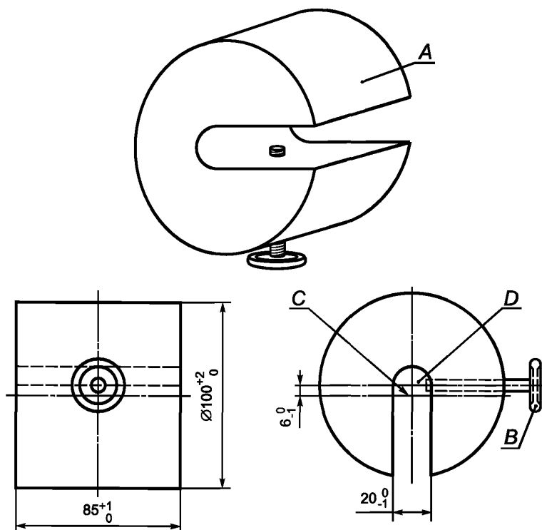
А — груз массой приблизительно 4,5 кг; В — крепежный винт; С — ось груза; D — ось крепежного винта
