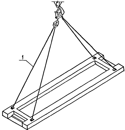
Схема строповки плиты перекрытия типа ПР
