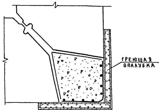
Отогрев и обогрев стыка в греющей опалубке
