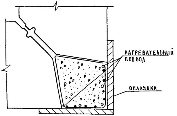
Обогрев стыка нагревательными проводами
