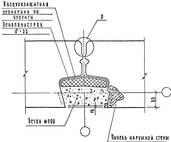
Вариант герметизации стыка отверждающейся мастикой
