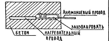
СОЕДИНЕНИЕ НАГРЕВАТЕЛЬНОГО ПРОВОДА
