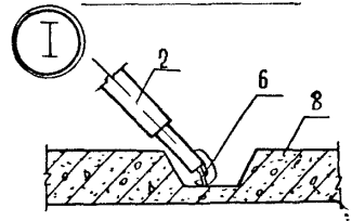
КРЕПЛЕНИЕ ПОДКОСА ЗА МОНТАЖНУЮ ПЕТАЮ ПЕРЕКРЫТИЯ
