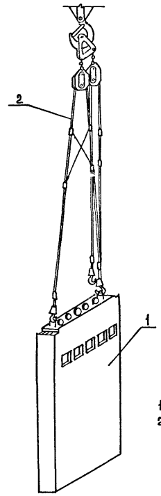
СХЕМА СТРОПОВКИ ВЕНТИЛЯЦИОННЫХ БЛОКОВ
