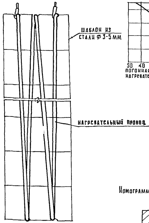
Шаблон с нагревательным проводом
