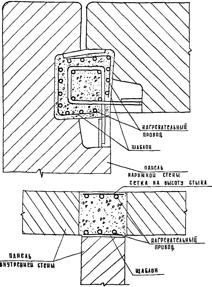
Шаблон с нагревательным проводом
