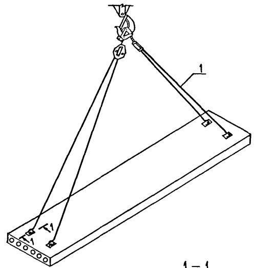
Схема строповки плиты перекрытия типа ПК
