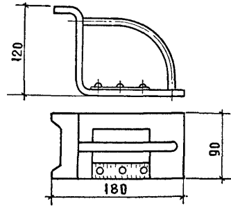
ШАБЛОН ДЛЯ УСТАНОВКИ НИЗА СТЕНОВЫХ ПАНЕЛЕЙ
