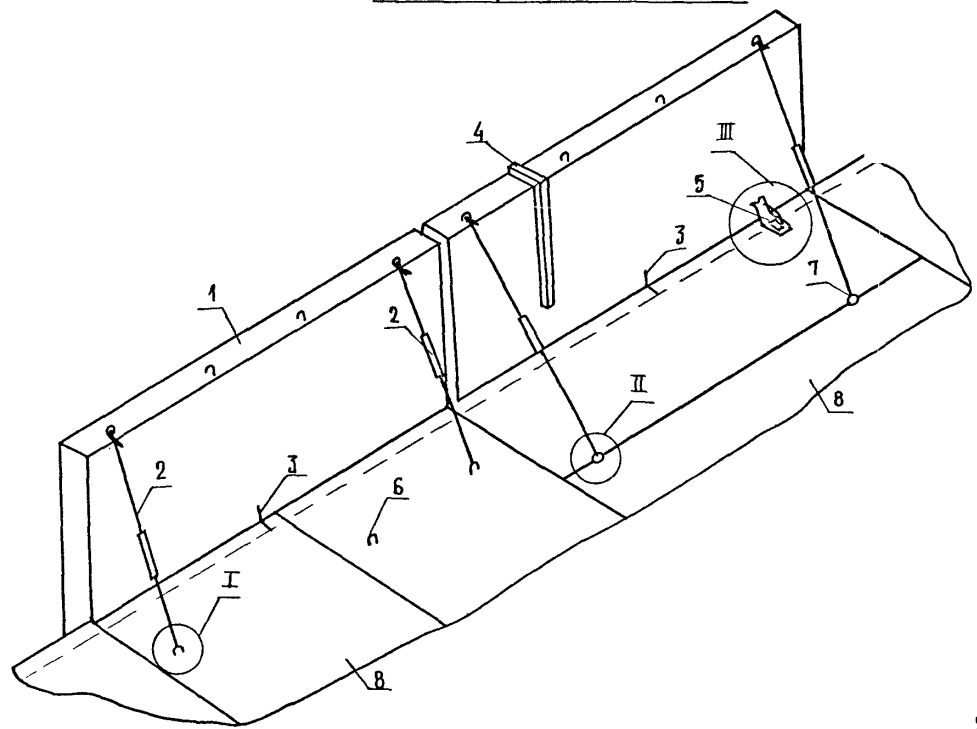
КРЕПЛЕНИЕ ПОДКОСА ЗА МОНТАЖНУЮ ПЕТАЮ ПЕРЕКРЫТИЯ
