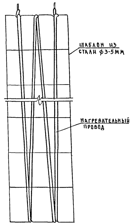
ШАБЛОН С НАГРЕВАТЕЛЬНЫМ ПРОВОДОМ
