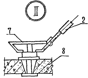
КРЕПЛЕНИЕ ПОДКОСА ЗА АНКЕР ЩЕЛЕВОЙ
