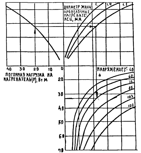
Монogramма для определения длины проводочных электронагревателей
