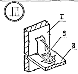
ВЫВЕРКА ПАНЕЛЕЙ В ПОПЕРЕЧНОМ НАПРАВЛЕНИИ С ПОМОЩЬЮ ШАБЛОНА
