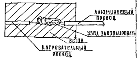
Соединение нагревательного провода с коммутирующим.
