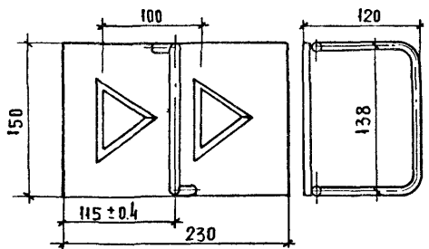
ШАБЛОН ДЛЯ РАЗБИВКИ РИСК
