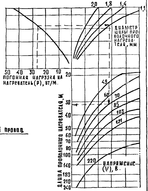
Нограмма для определения длины нагревателя
