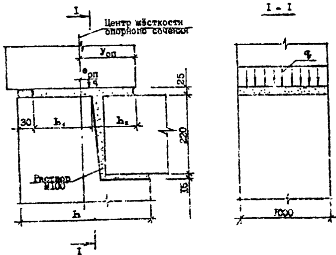
Расчетная схема стика
