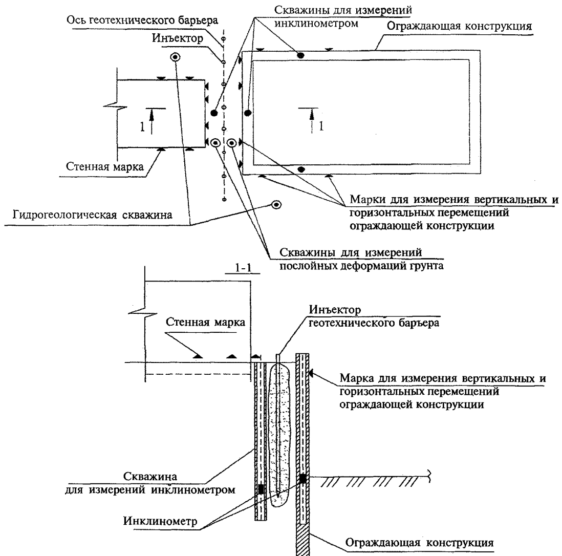
Рисунок 6.1 — Примерная схема расположения марок и скважин при проведении мониторинга (в случае устройства котлована)
