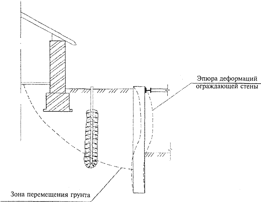
Рисунок 1.1 — Защита фундамента здания при устройстве котлована
