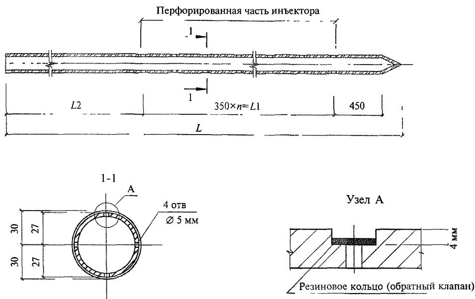
Рисунок 4.2 — Конструкция иньектора
