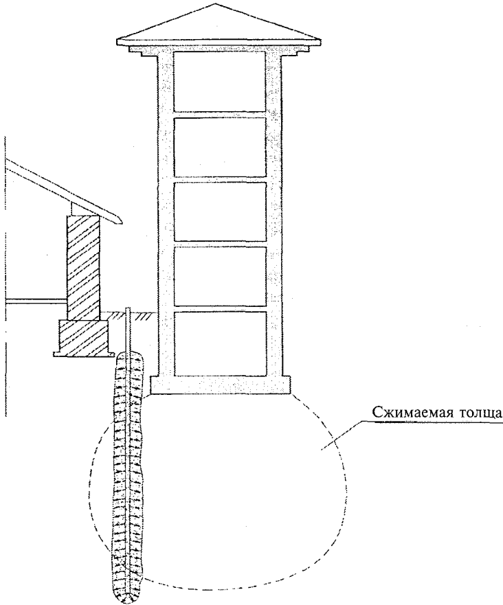
Рисунок 1.2 — Защита фундаментов существующего здания для снижения взаимного влияния фундаментов
