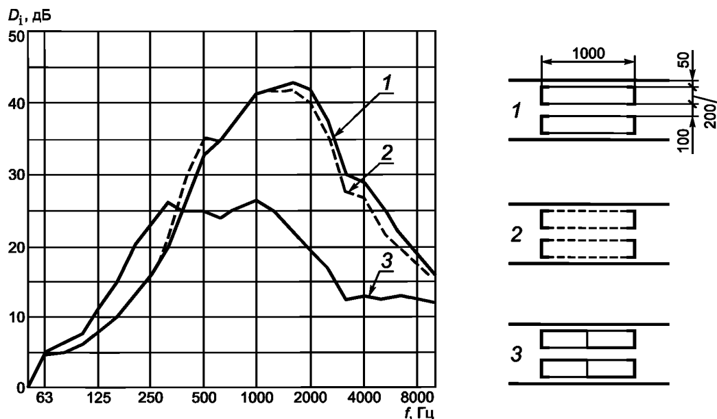
Рисунок 7 — Зависимость удельных потерь распространения D_a от частоты f для глушителя с пластинами разной толщины и ширины воздуховодов между пластинами, равной толщине пластин
