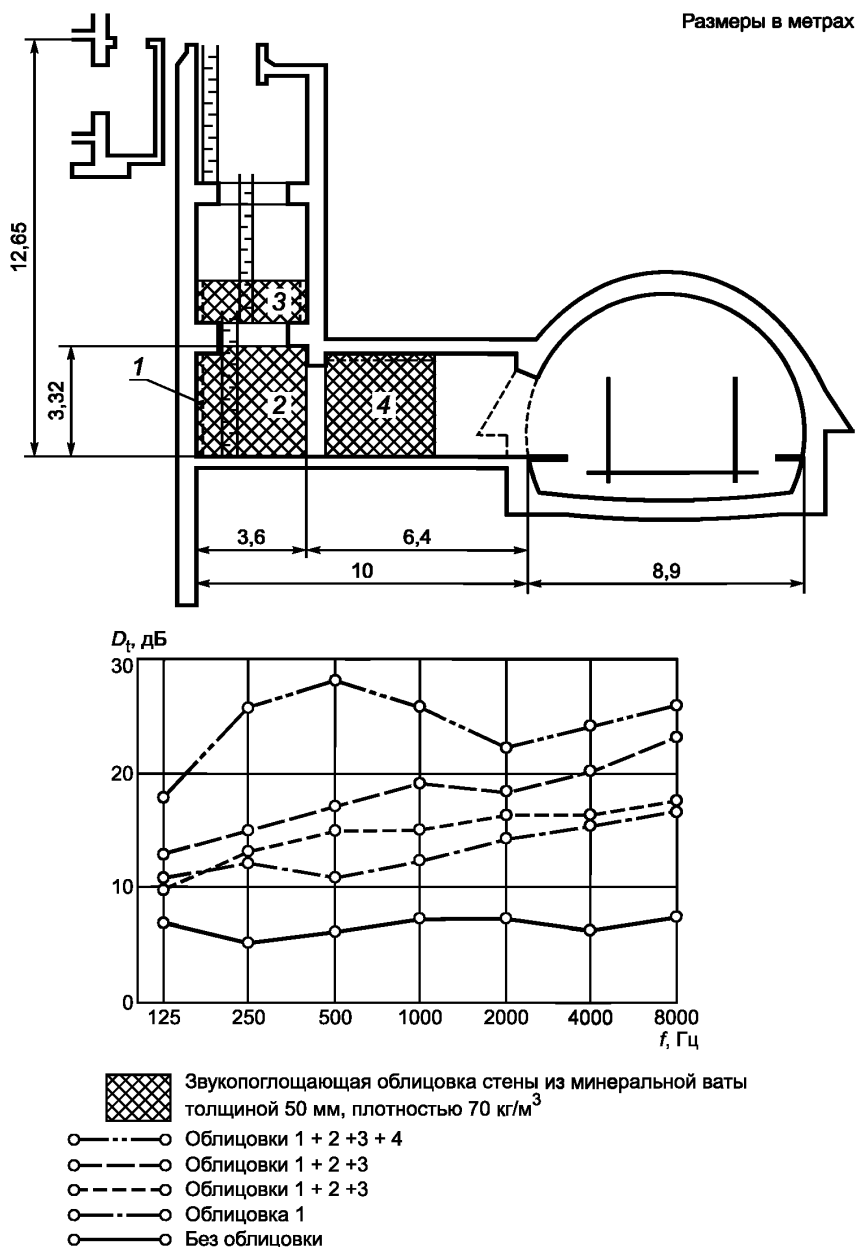
Рисунок 12 — Зависимость потерь при прохождении D_t от частоты f для поворота (изгиба) канала при различных способах размещения звукопоглощающей облицовки стенок (вентиляционная шахта подземного туннеля)
