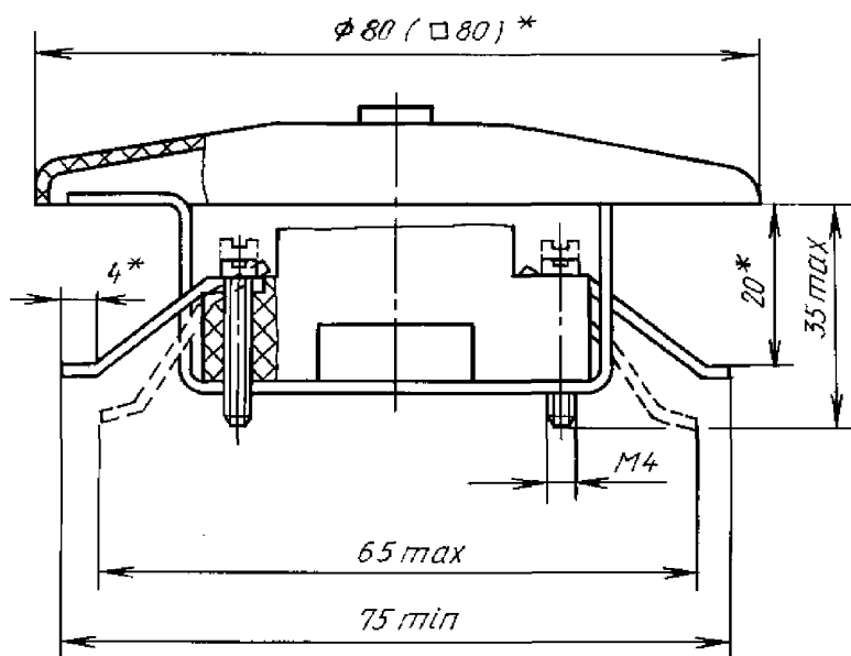
а) выключатель для скрытой установки
