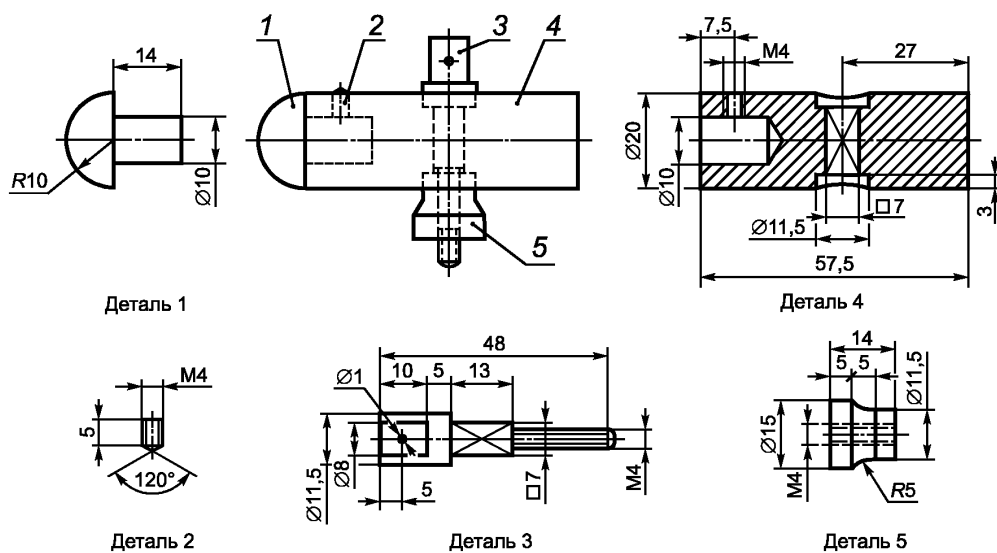
Рисунок А.19 — Устройство для испытания на удар
