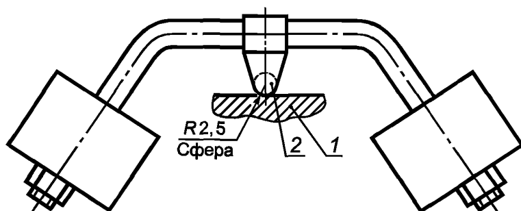
1 — образец; 2 — стальной шарик диаметром 5 мм
