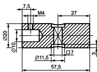
Рисунок А.19 — Устройство для испытания на удар
