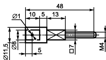
Рисунок А.20 — Устройство маятника для испытания на удар
