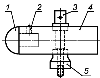
Рисунок А.19 — Устройство для испытания на удар
