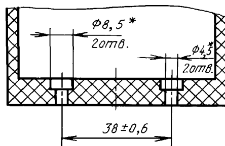
б) установочные размеры выключателей степени защиты IP20
