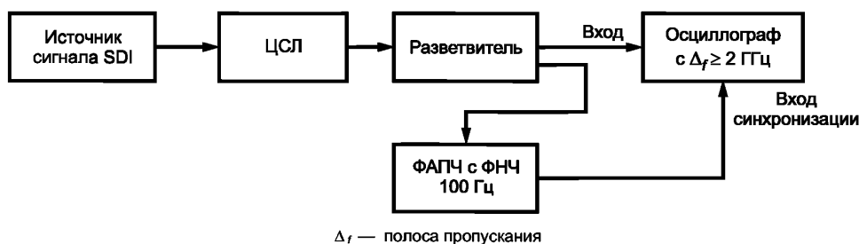
Рисунок 9 — Схема измерения высокочастотного фазового дрожания цифрового сигнала
