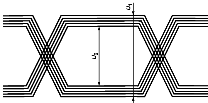
Рисунок 7 — Диаграмма, поясняющая измерение дрожания уровня цифрового сигнала
