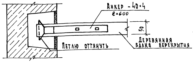
ФРАГМЕНТ ПЛАНА ДЕРЕВЯННОГО ЦИТОВОГО ПЕРЕКРЫТИЯ
