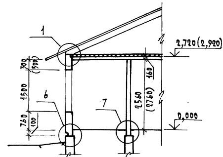
1-1 ОДНОЭТАЖНЫЙ ДОМ
