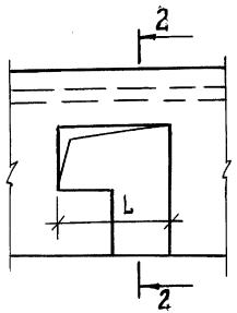
ЭЛЕМЕНТЫ ОБРАМЛЕНИЯ БАЛКОННОГО ПРОЕМА
