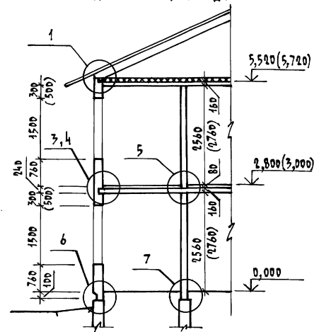
1-1 ОДНОЭТАЖНЫЙ ДОМ
