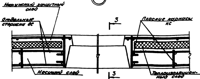
Деталь наружной трехслойной стены с оконным проемом
