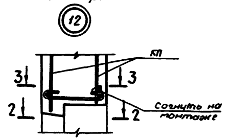
Деталь наружной однослойной стены с оконным проемом
