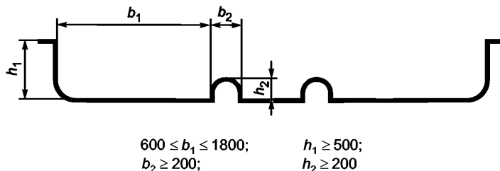
Рисунок 8 — Поперечное сечение горки типа 6
