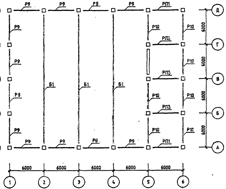
МОНТАЖНЫЙ ПЛАН РИГЕЛЕЙ И СВЯЗЕВЫХ ПЛИТ ОТМ. +6.50 ( +9.80 )
