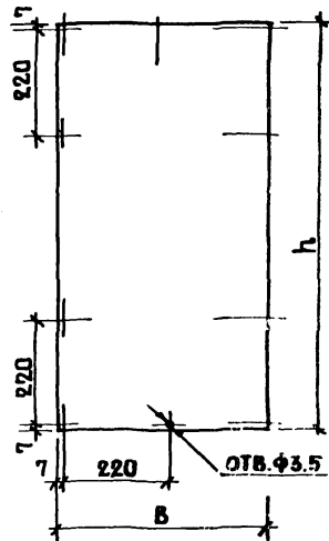
РИС. 2 ОСТАЛЬНОЕ СМ.РИС.1
