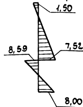
Эпюра поперечных сил в тс/м
