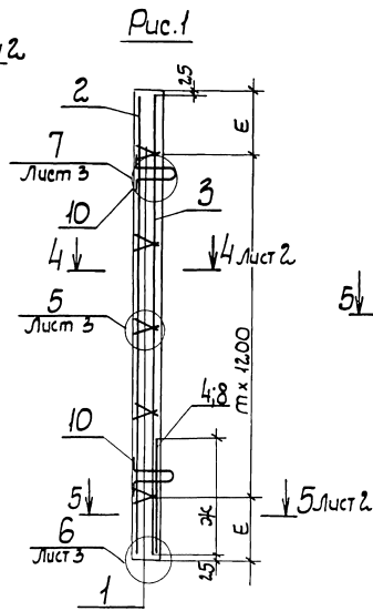
Таблицы исполнений см. лист 4;5.
