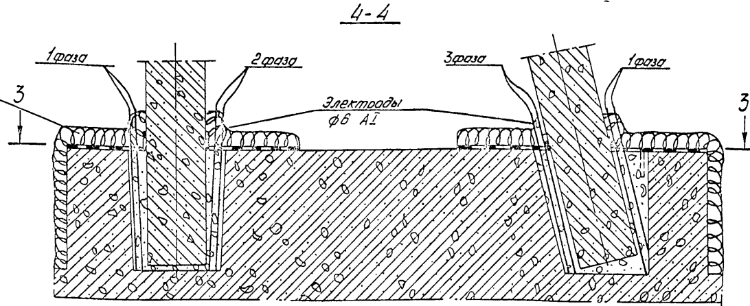
Стыки стоек в стаканах фундамента
