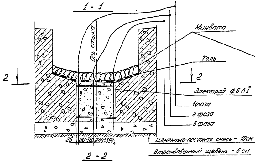
Стык блоков фундамента
