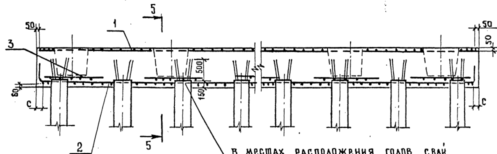
Армирование 4-4
