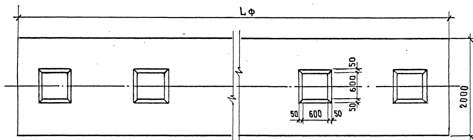
Армирование 4-4
