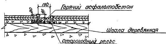
Детали укладки асфальтобетонного покрытия с внутренней стороны колеи
