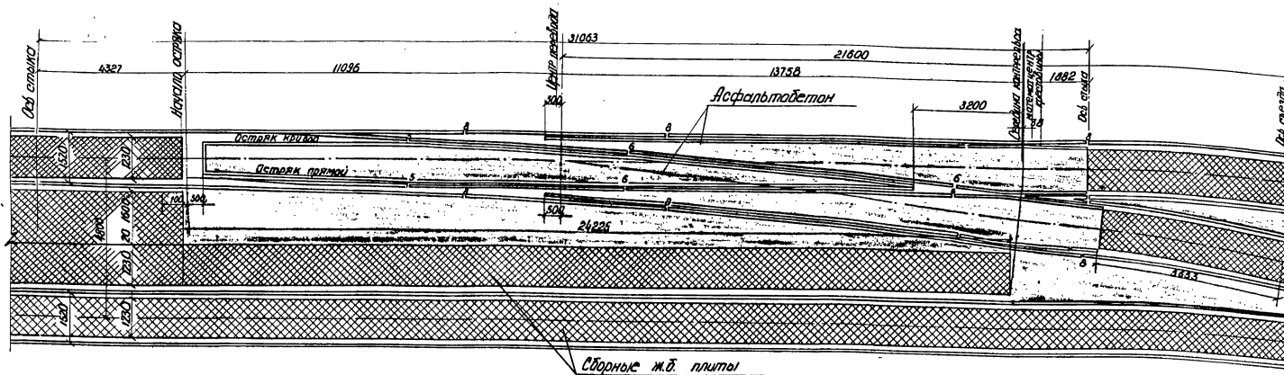
Детали укладки асфальтобетонного покрытия с внутренней стороны колеи
