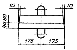
Вид 3-3
