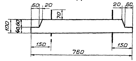
ПЛАН
