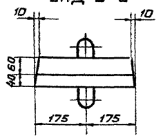
Вид 3-3
